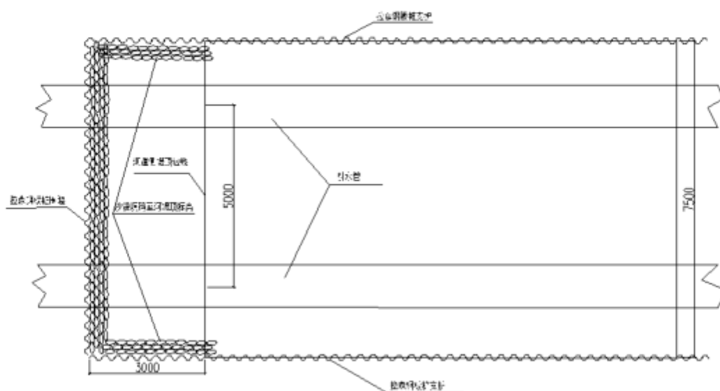
图 3.3-11 基坑开挖支护及河道围堰平面图
