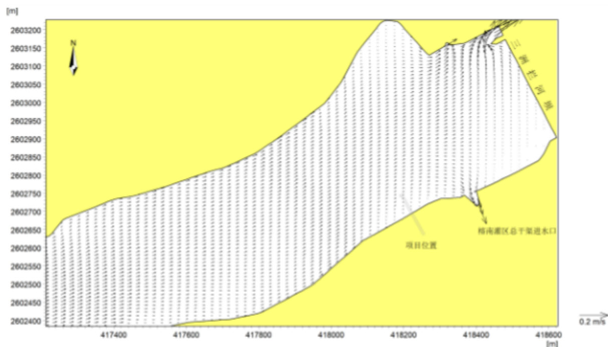
图 5.2-5 项目附近河段流场图
