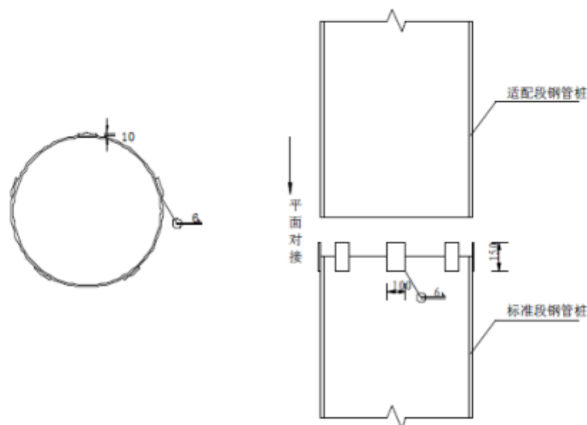
图 3.3-6 钢管桩对接焊接示意图
