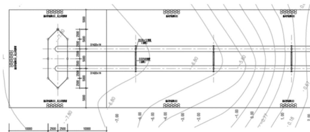
图 3.3-10 抛石护底区域
