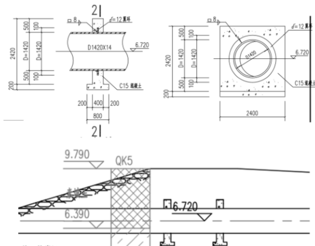
图 3.3-12 止水墙构造及布置图
