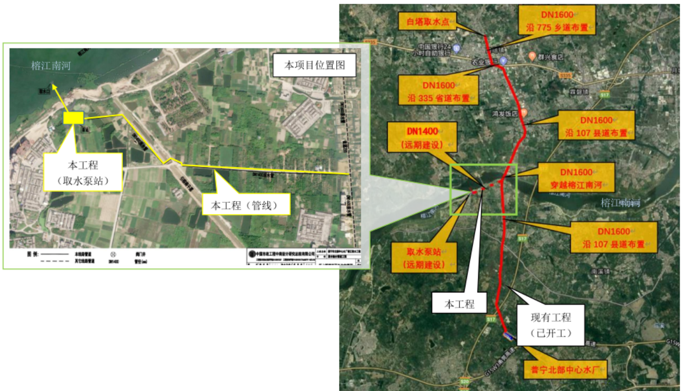
图 1.1-2 本项目工程内容示意图
