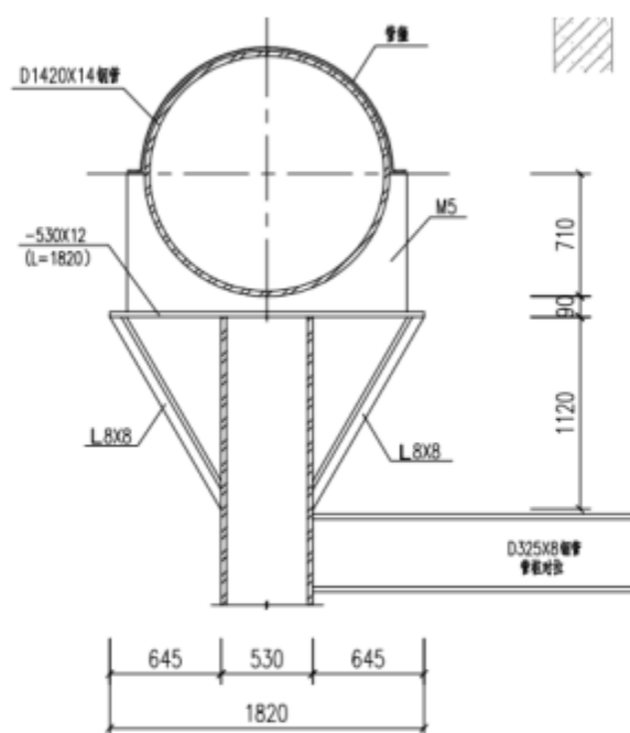
图 3.3-7 钢管桩桩顶构造图
