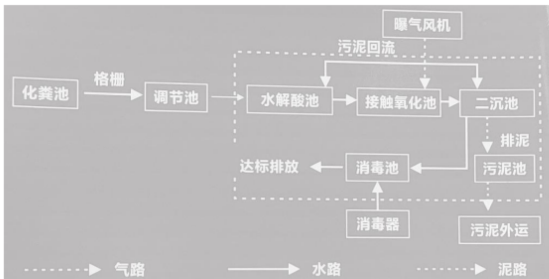
图 6.2-2 污水处理设施工艺图
