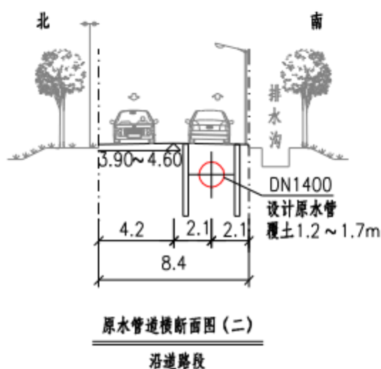
图 3.3-5 原水管道（沿道路）铺设横断面布置图
