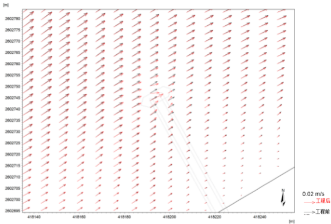
图 5.2-11 工程前后的取水口附近局部水域的流场对比图
