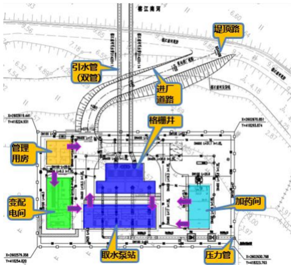
图 3.3-3 取水泵站平面布置图
