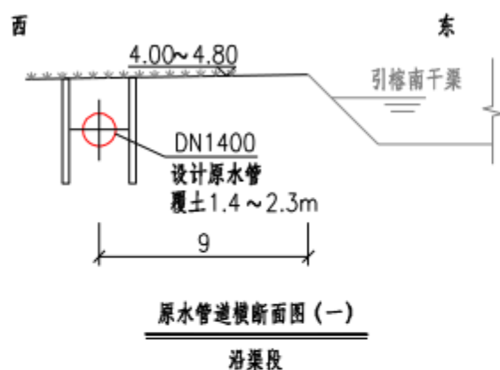
图 3.3-4 原水管道（沿引榕南干渠）铺设横断面布置图
