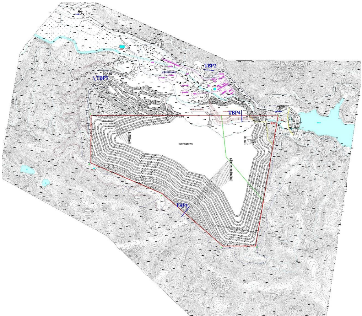
图 3-1 土质边坡分布位置示意图
