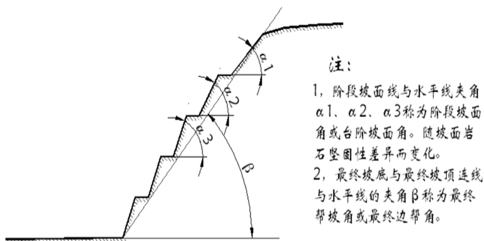
图 1-4 最终边帮构成要素图
