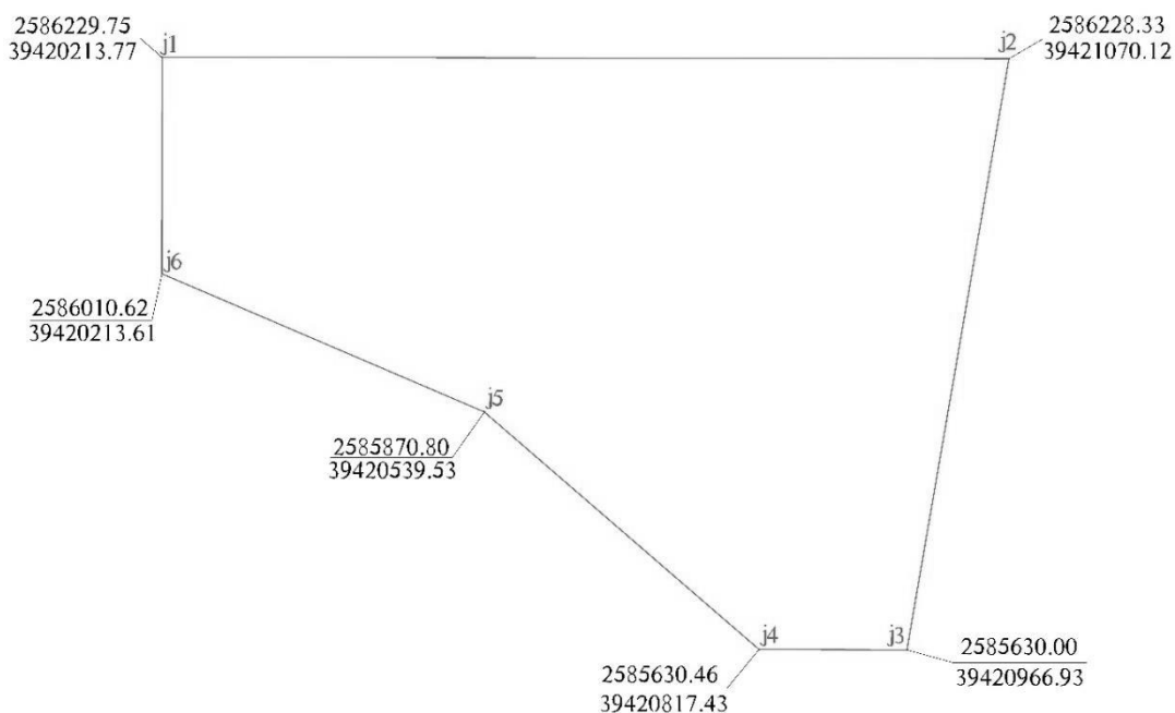
图 1-2 矿区范围示意图
