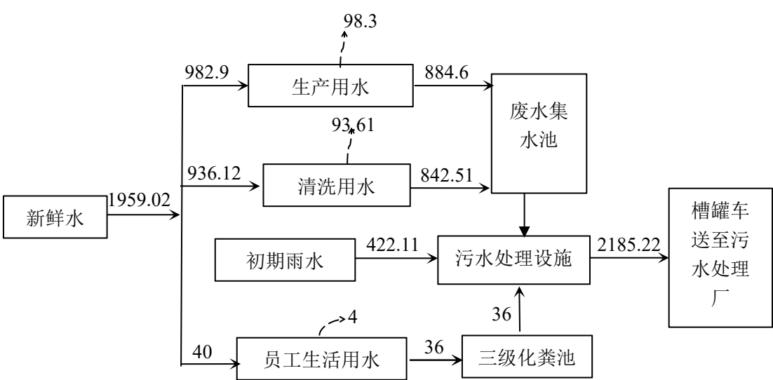
图 2-1 项目总水平衡图 (t/a)
