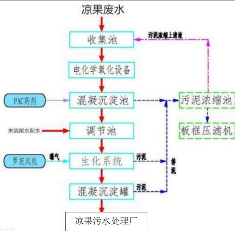
图 4-1 项目废水处理工艺流程图
