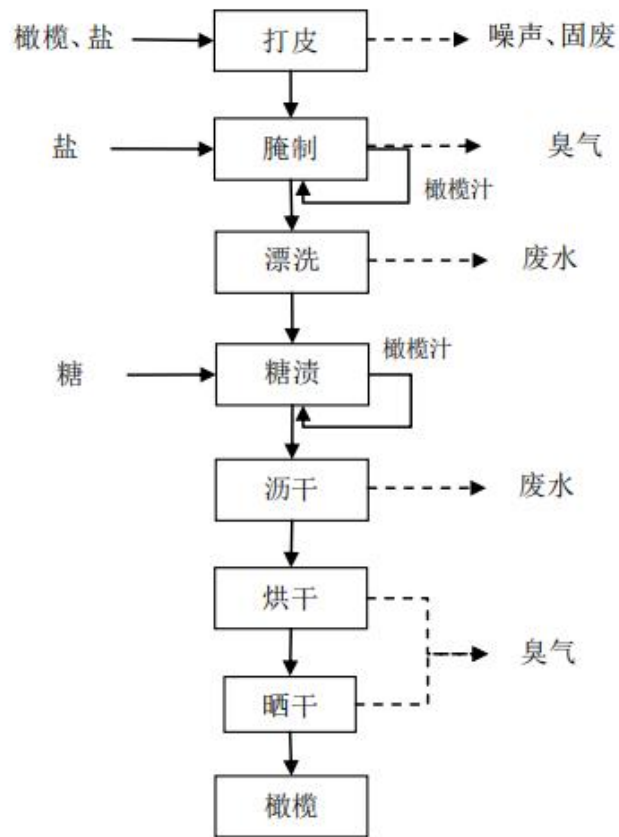
图2-2 橄榄蜜饯生产工艺流程及产污环节图
