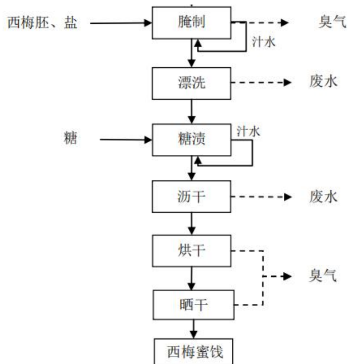
图2-3 西梅蜜饯生产工艺流程及产污环节图
