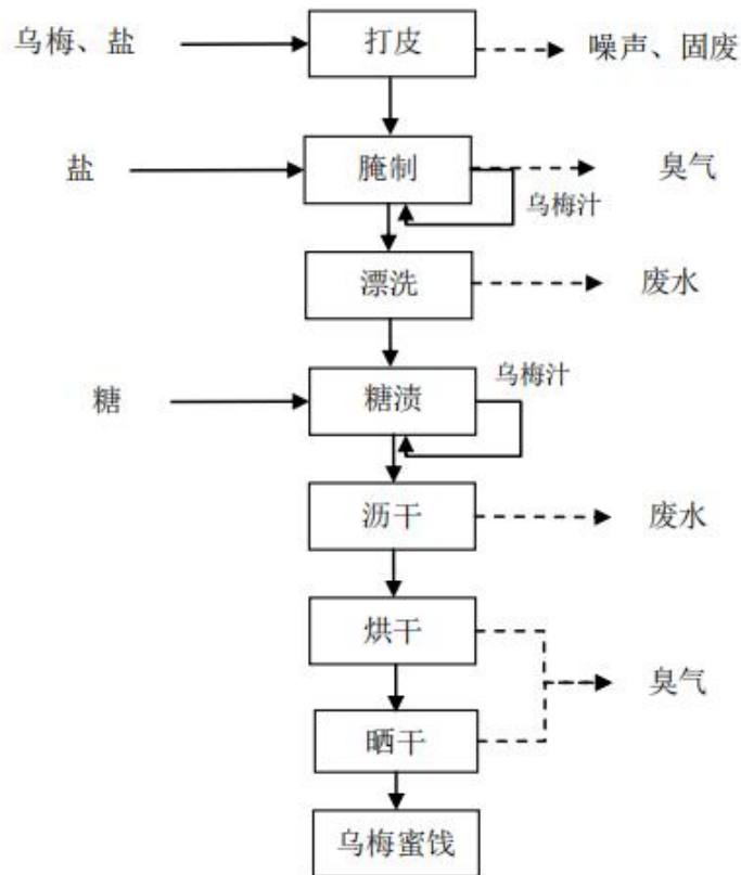
图2-6 乌梅蜜饯生产工艺流程及产污环节图
