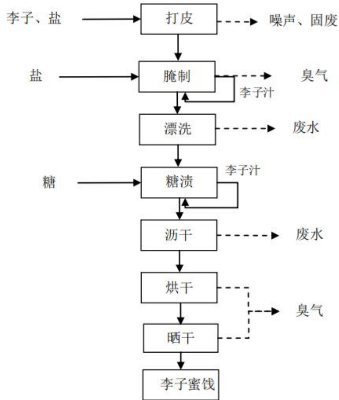
图2-5 李子蜜饯生产工艺流程及产污环节图
