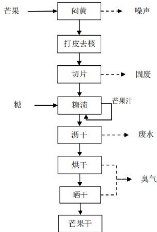
图2-4 芒果干生产工艺流程及产污环节图
