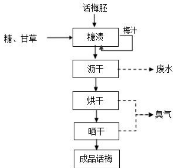
图 2-6 项目话梅生产工艺流程图
