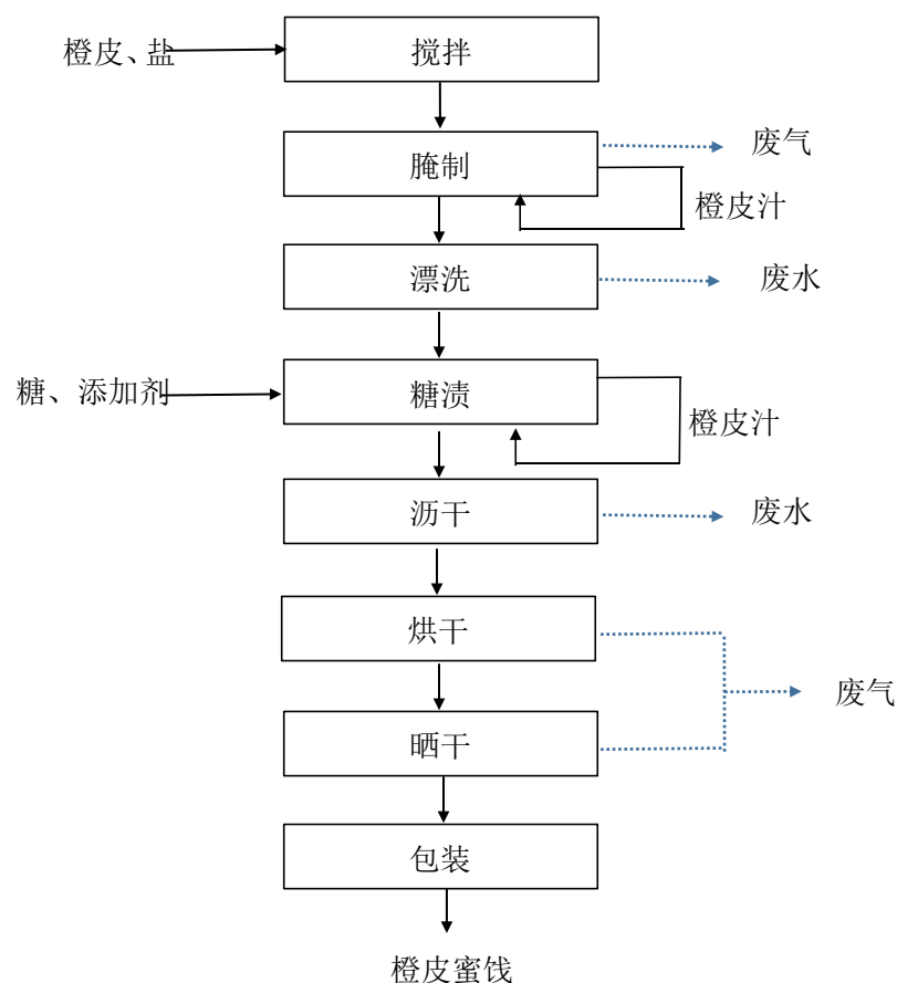
图2-2 橙皮蜜饯生产工艺流程及产污环节图
