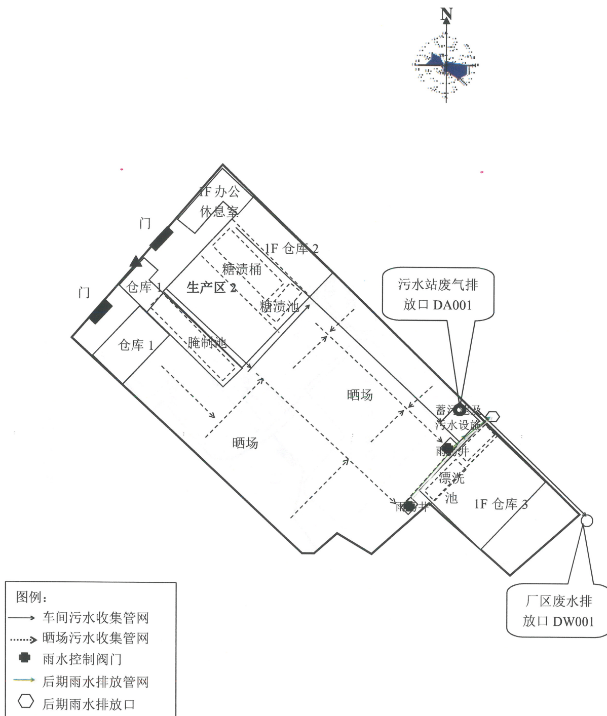
附图 3-2 项目厂区二平面布置图
