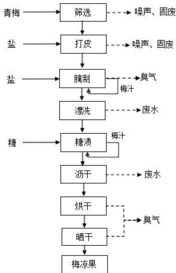
图 2-3 项目梅凉果生产工艺流程图
