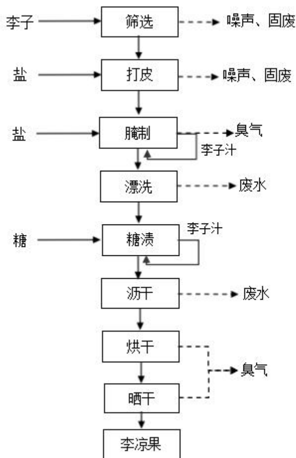
图 2-4 项目李凉果生产工艺流程图
