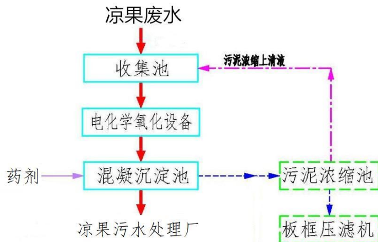
图 4-1 项目废水处理工艺流程图
