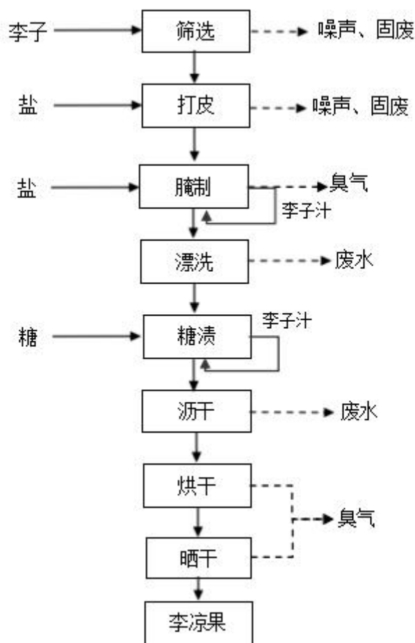
图 2-2 项目李凉果生产工艺流程图
