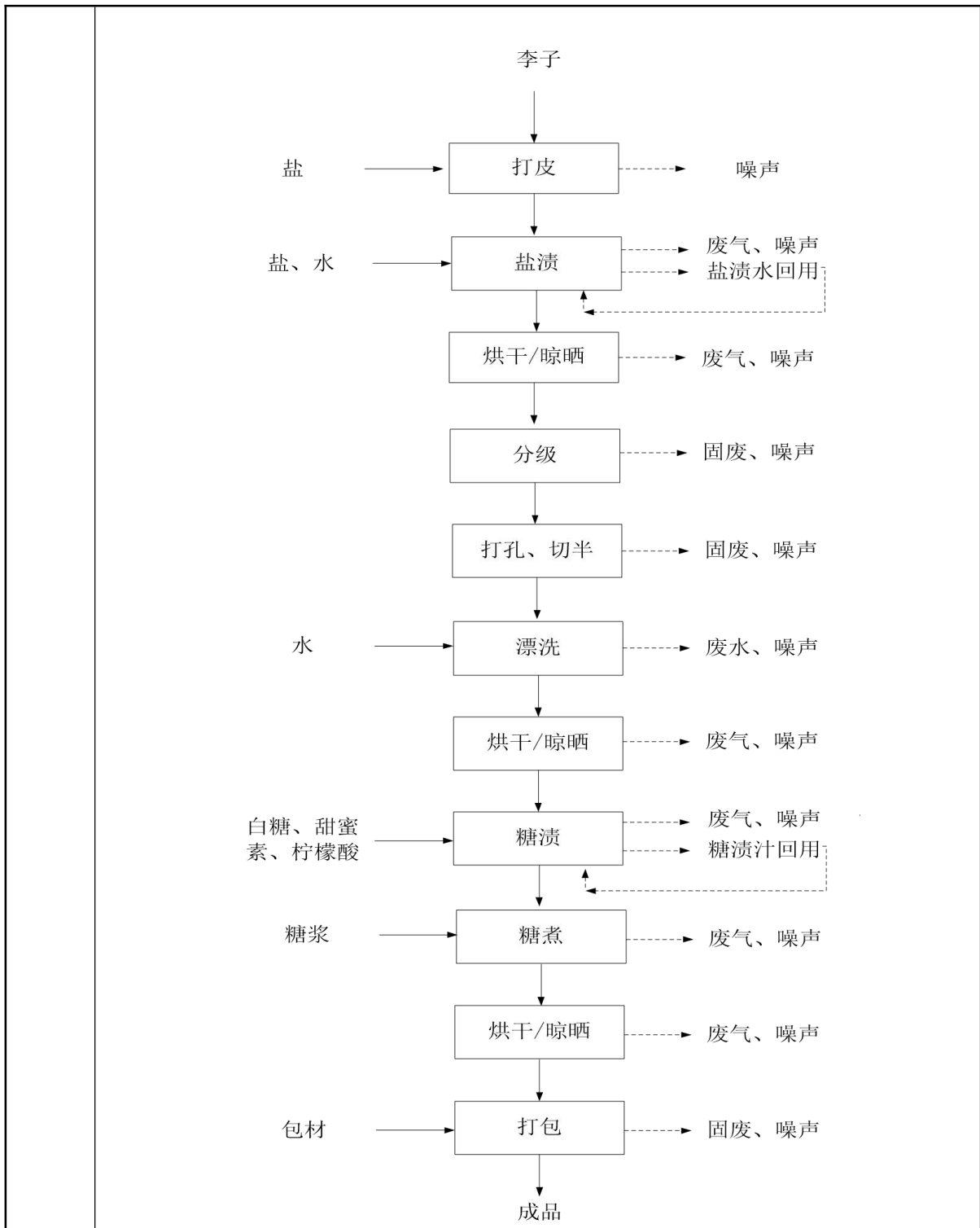
图 2-2 李子生产工艺流程图
