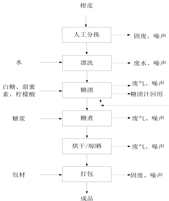
图 2-4 柑皮生产工艺流程图
