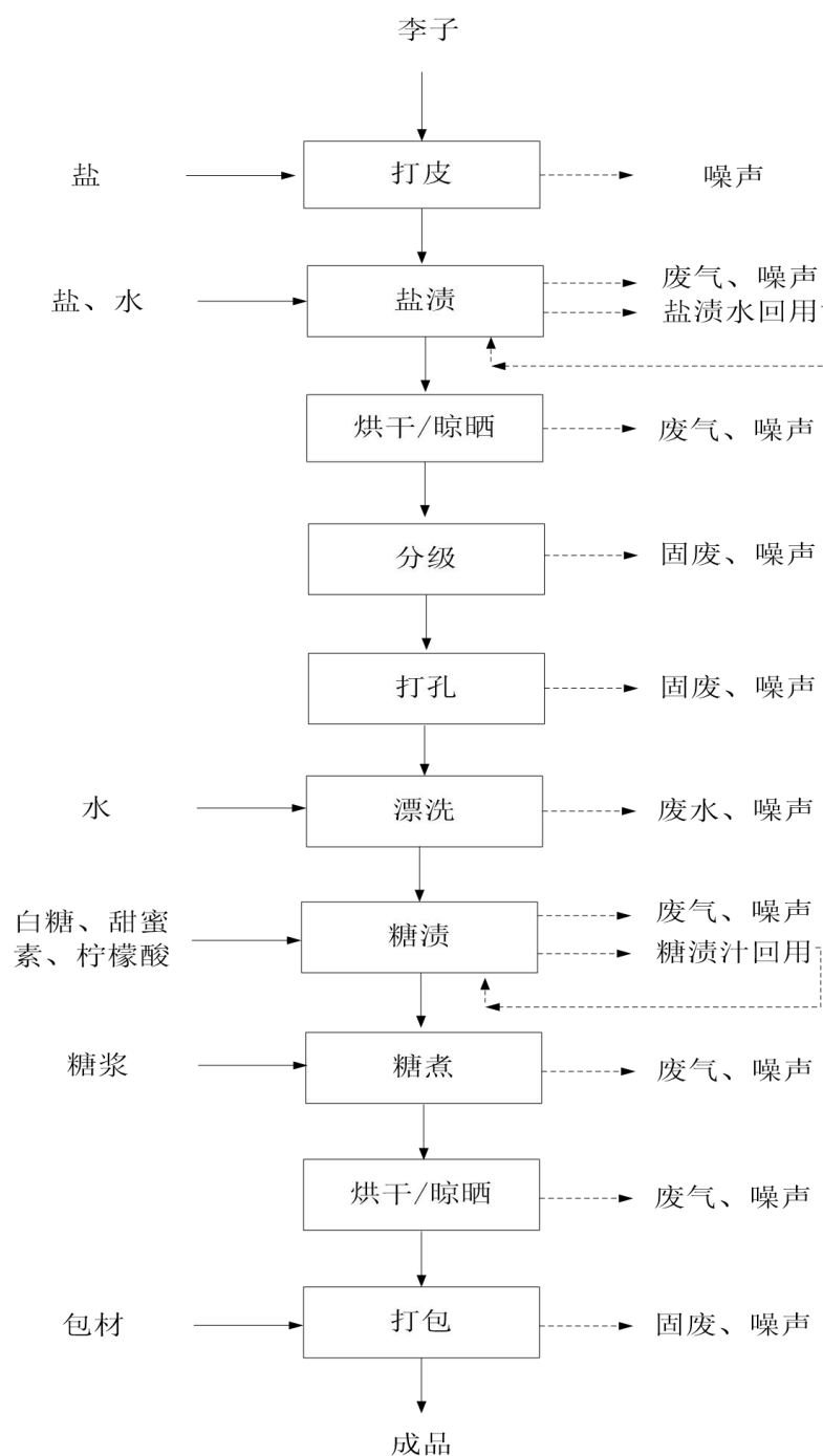
图 2-2 李子生产工艺流程图
