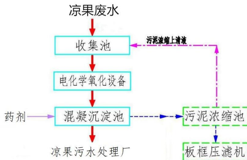
图 4-1 厂内污水处理站废水预处理工艺流程图
