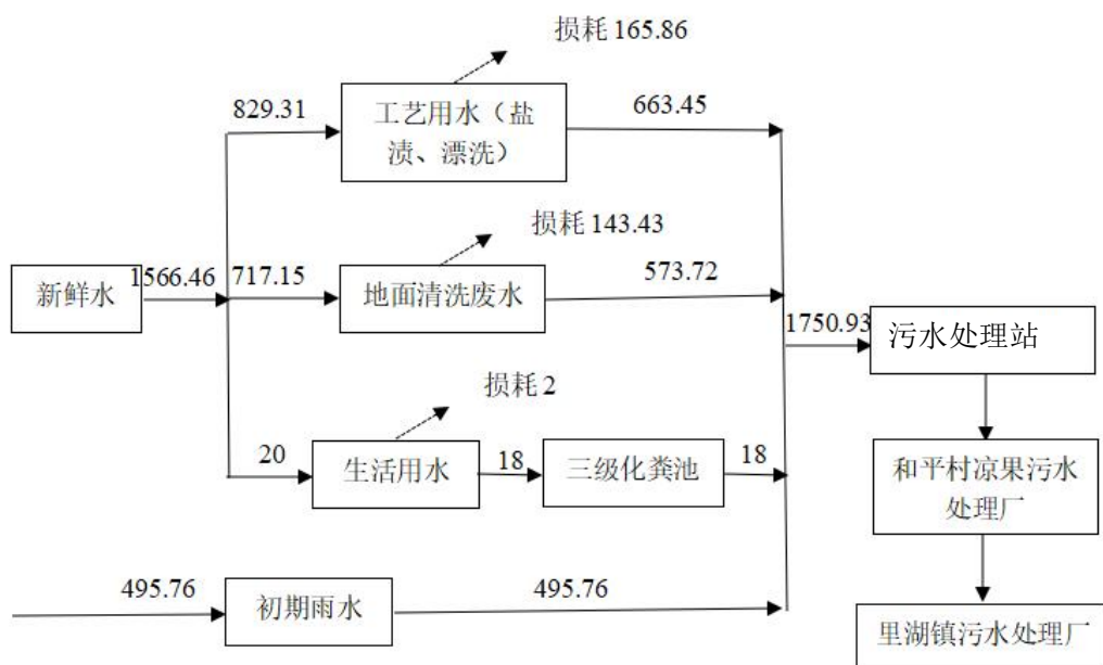
图 2-1 项目用水平衡示意图（单位：t/a）
