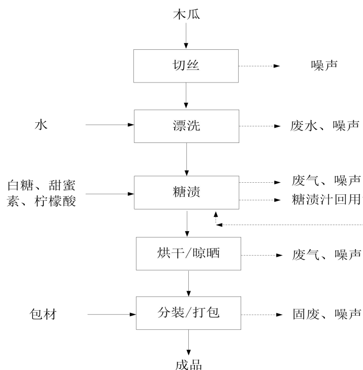
图 2-3 木瓜丝生产工艺流程及产污环节图
