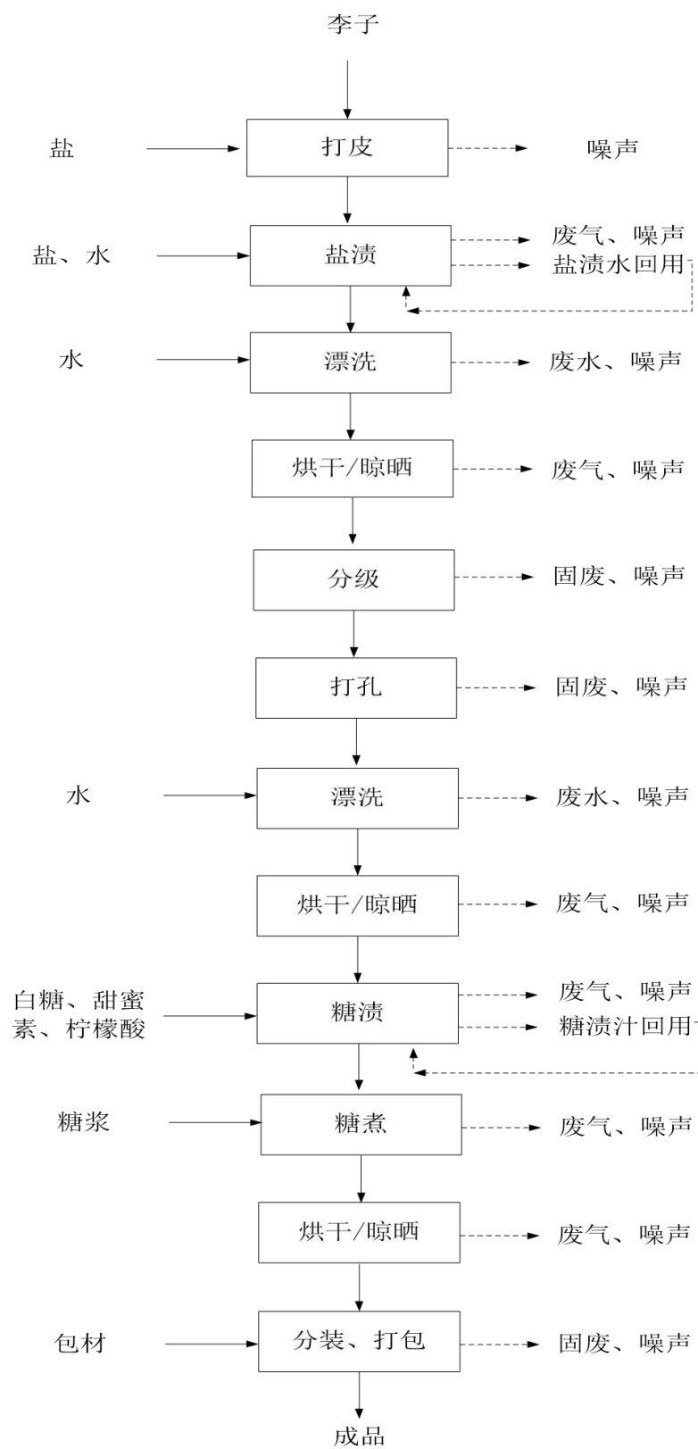
图 2-2 李子生产工艺流程图
