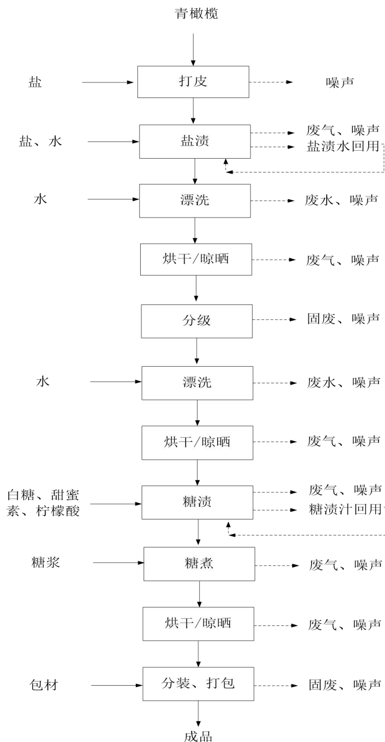
图 2-4 青橄榄生产工艺流程图
