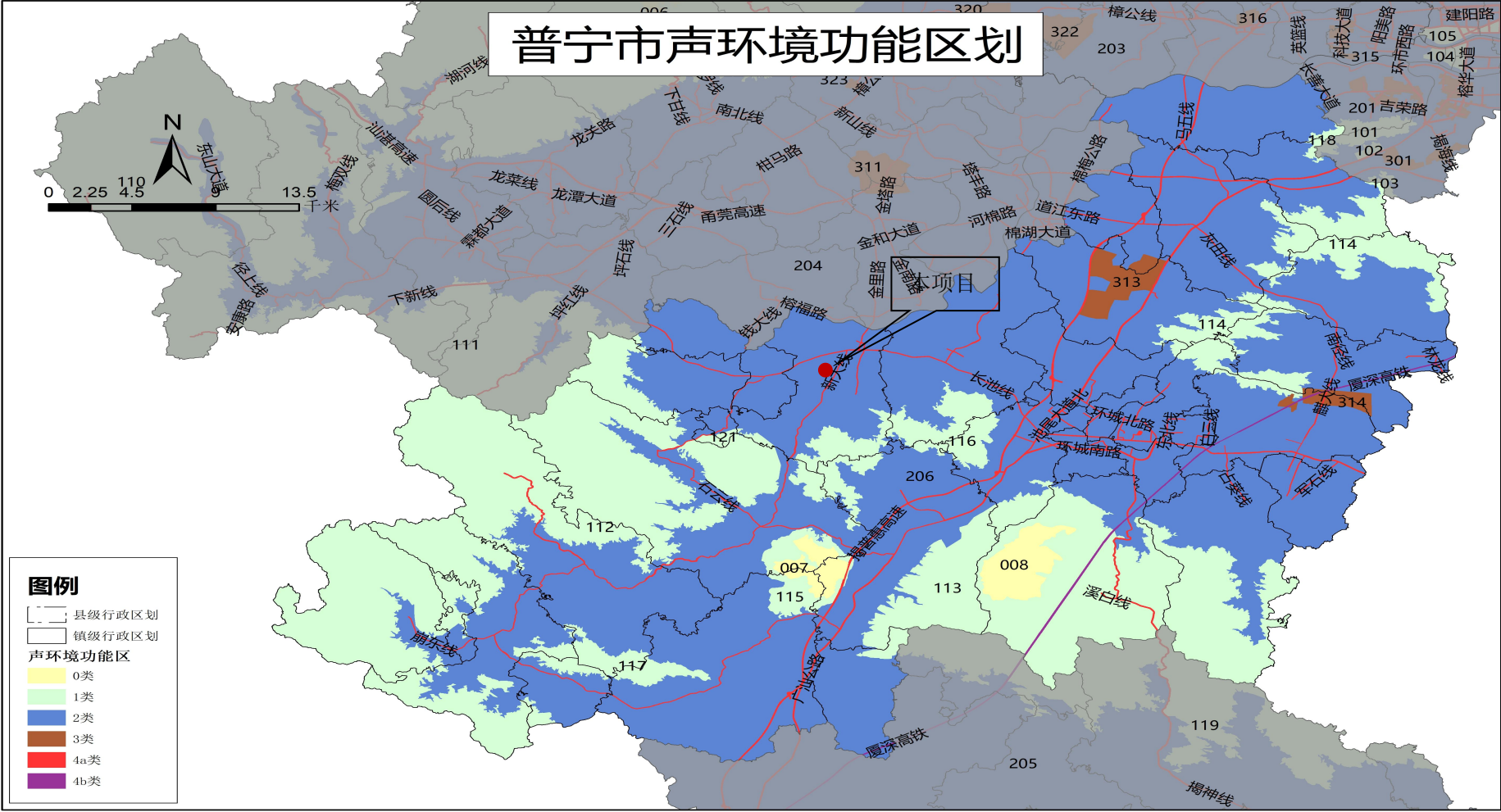
附图 14：普宁市区域环境噪声功能区划图
