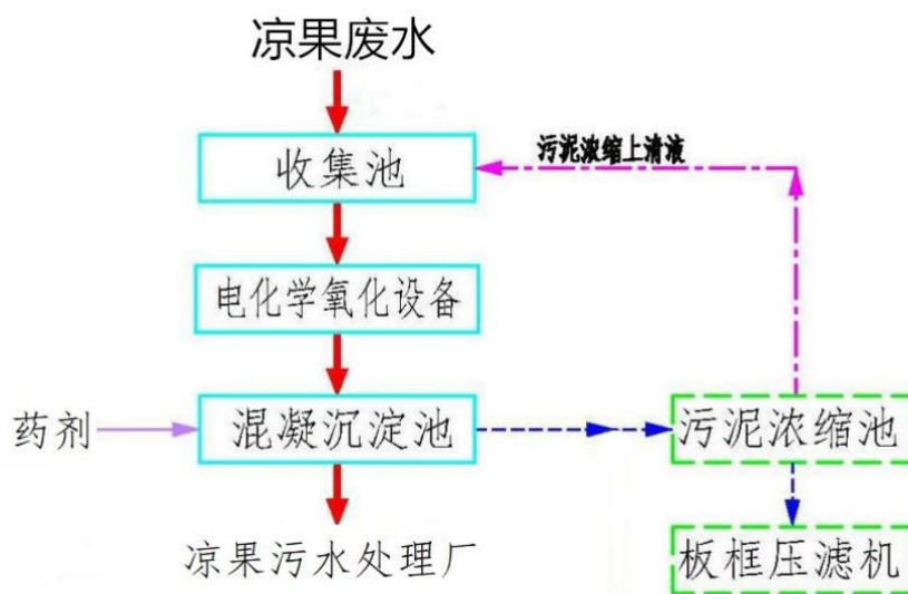
图 4-1 厂内污水处理站废水预处理工艺流程图
