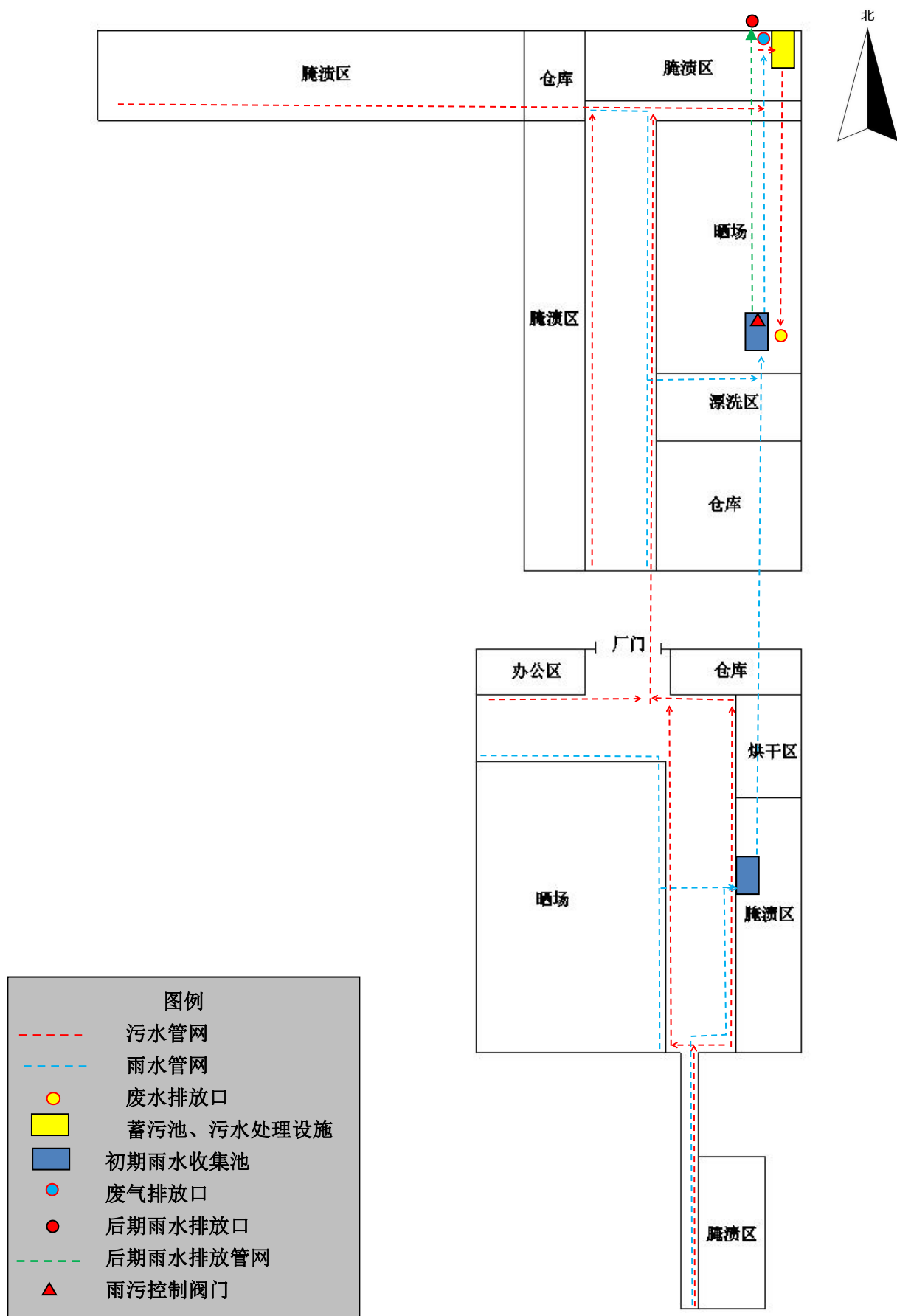
附图 5 本项目平面布置图
