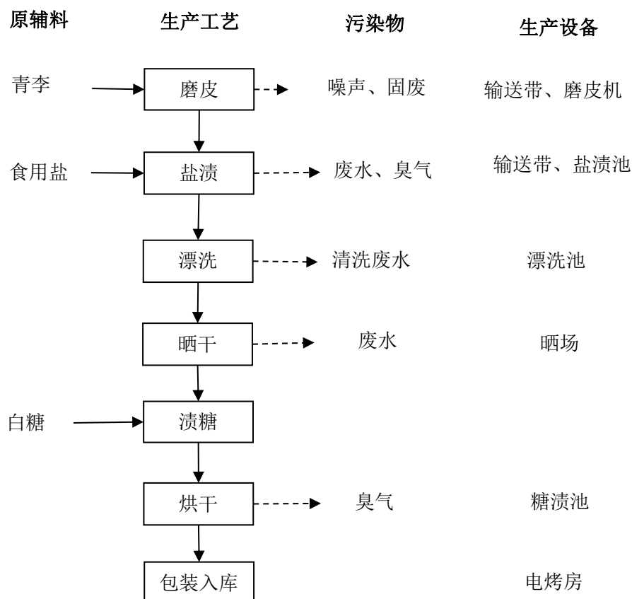
图 2-1 青李加工工艺流程及产污环节
