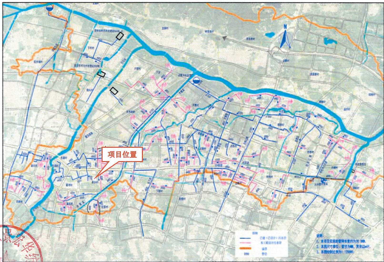
附图 7 占陇镇污水处理厂纳污范围图
