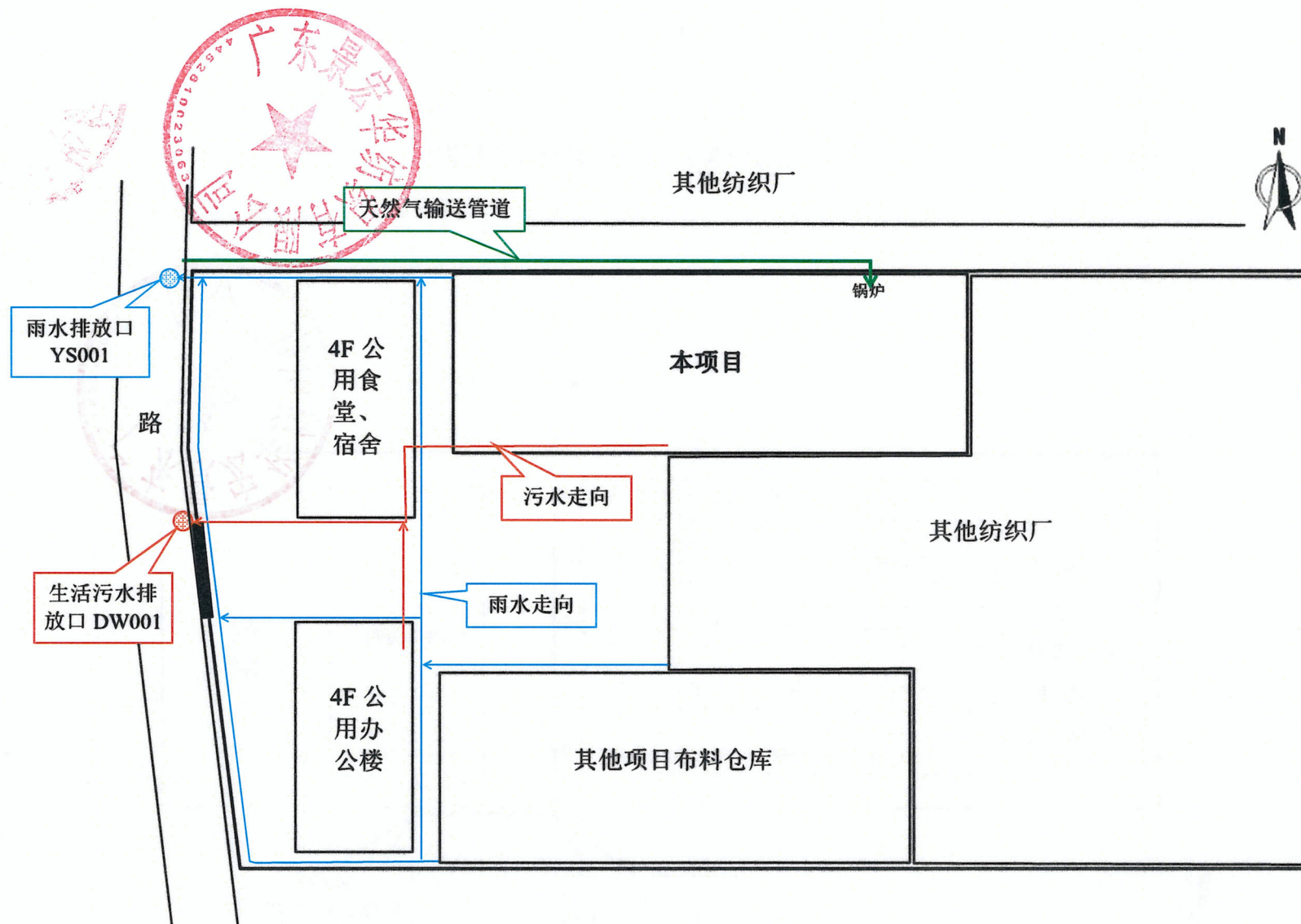
附图 4 项目天然气管道及生活污水排放管线图
