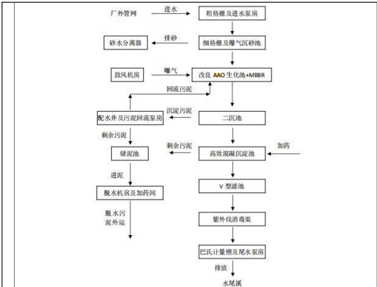
图 4-2 普宁市占陇污水处理厂污水处理工艺
