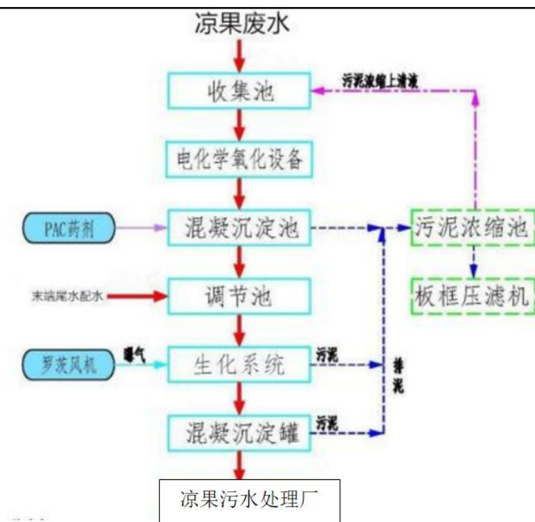
图 4-1 项目废水处理工艺流程图
