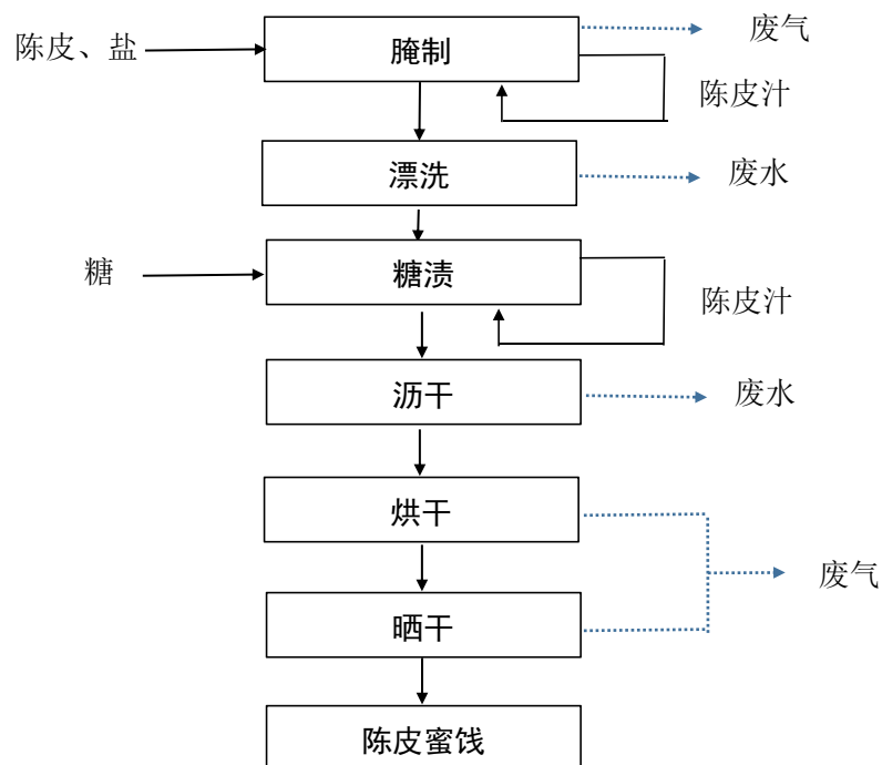
图2-4 陈皮蜜饯生产工艺流程及产污环节图
