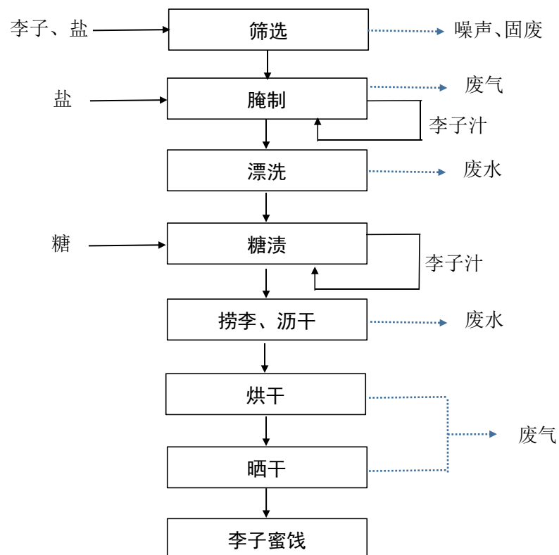
图2-2李子蜜饯生产工艺流程及产污环节图
