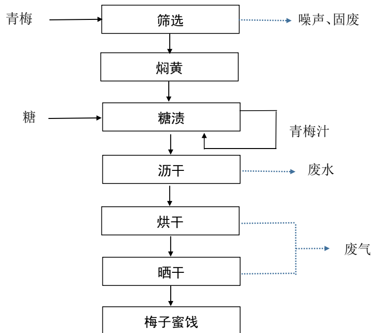
图2-3 梅子蜜饯生产工艺流程及产污环节图
