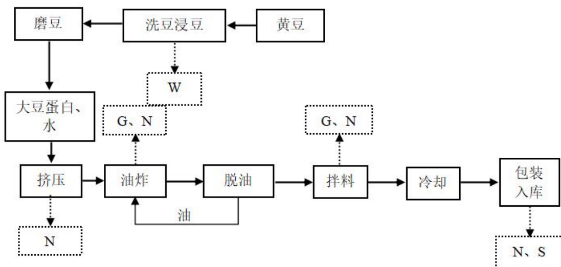
图 2-4 豆制品生产工艺流程及产排污环节图
