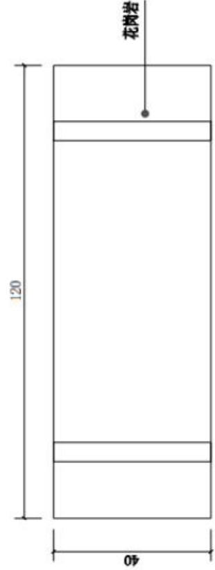
石凳平面图 1:10
