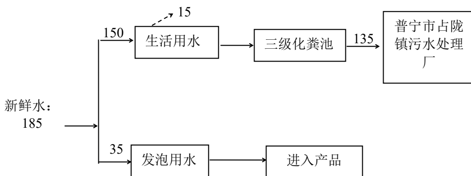
图 2-1 全厂用排水平衡图（单位：m³/a）
