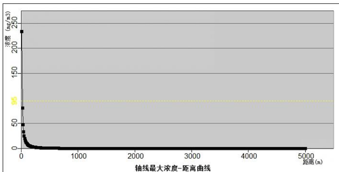
图7-5 火灾、爆炸次生/伴生HCN轴线的最大浓度图
