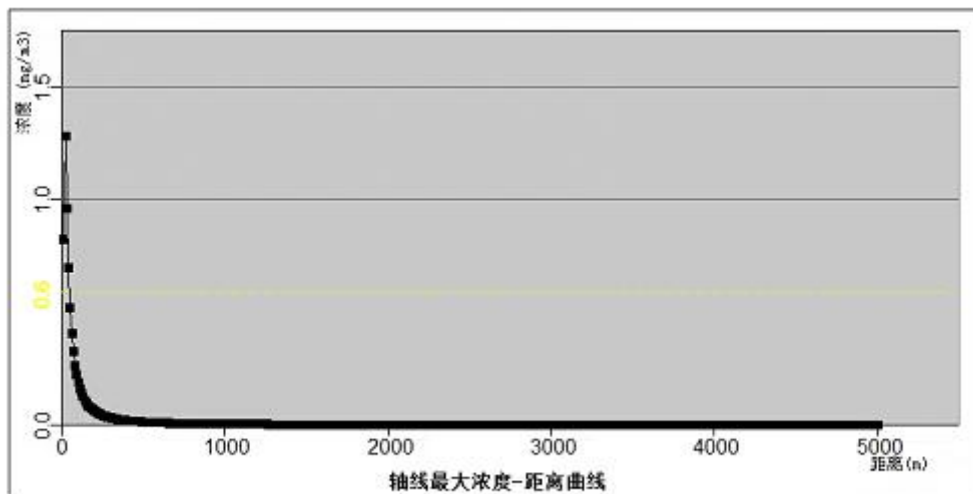
图7-1 TDI泄漏事故排放预测因子轴线的最大浓度图
