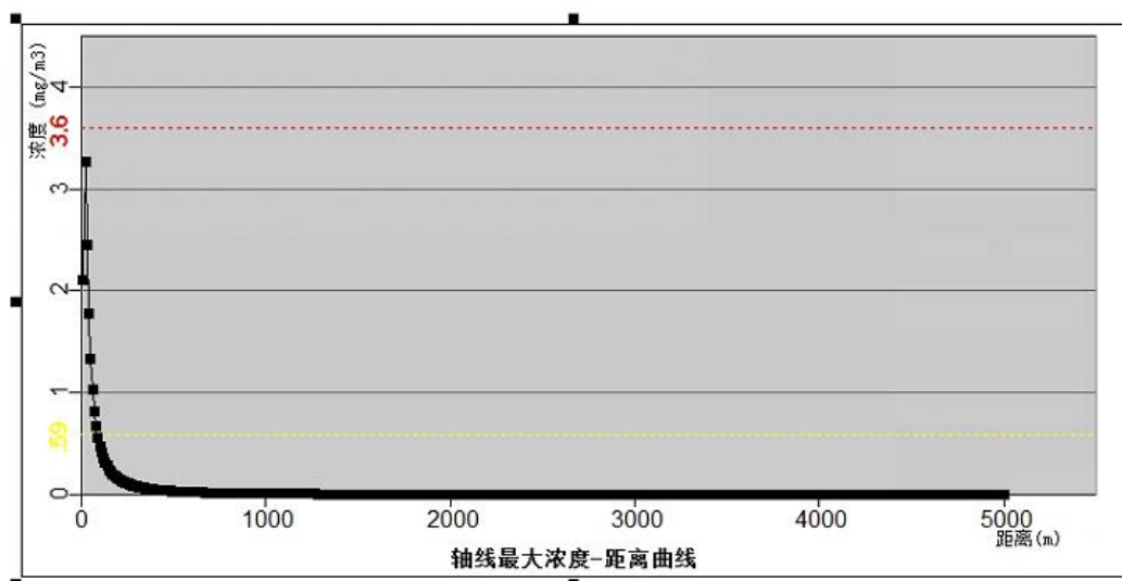
图7-2 TDI泄漏火灾、爆炸事故排放预测因子轴线的最大浓度图
