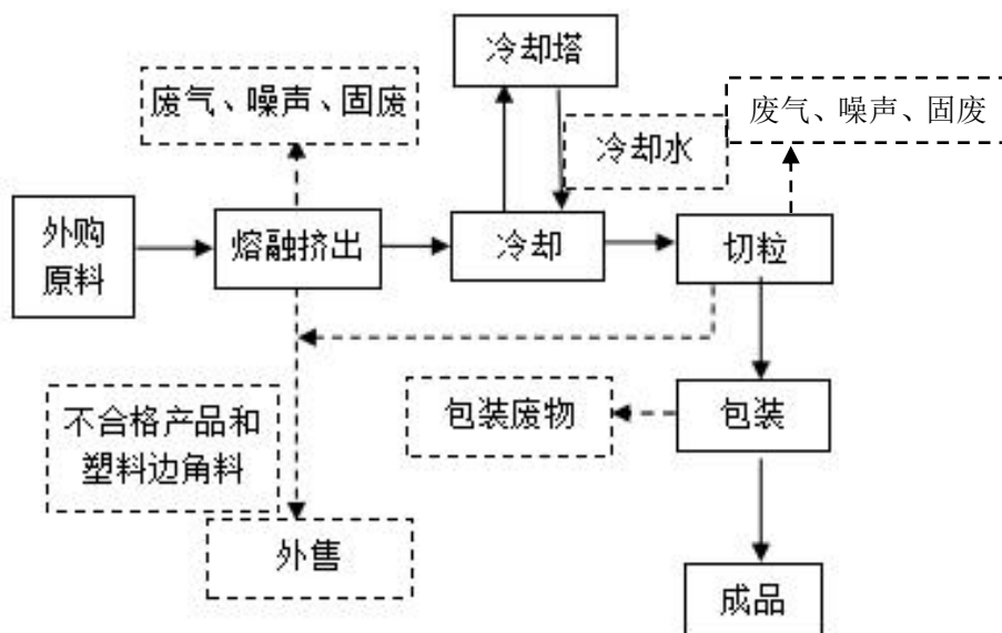
图 2-2 项目生产工艺流程及产排污环节图
