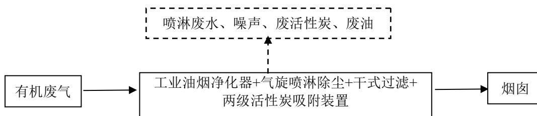
图 2-3 项目废气处理工艺流程及产污环节图
