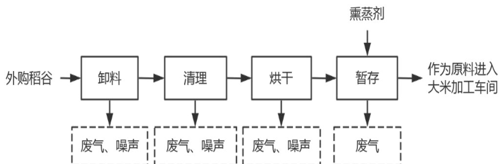
图 2-3 稻谷烘干工艺流程及产污环节图
