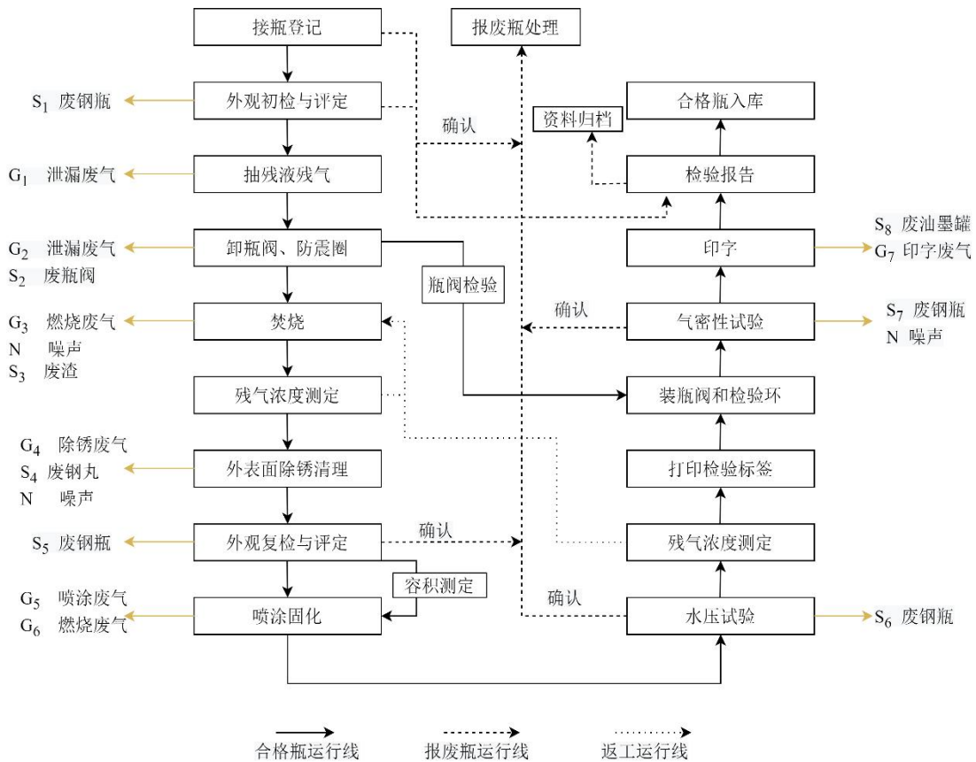
图2-2项目生产工艺及产污环节图
