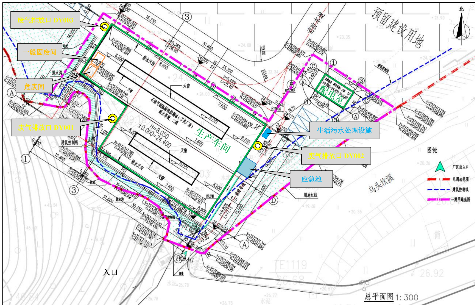
附图 6 项目总平面布置图
