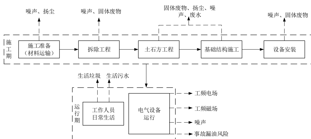
图 2-1 工艺流程及产污环节图
