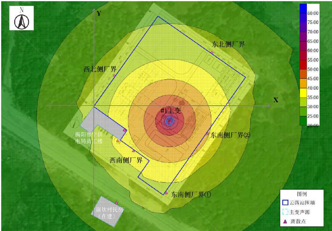
图 4-1 噪声贡献值等声值线图
