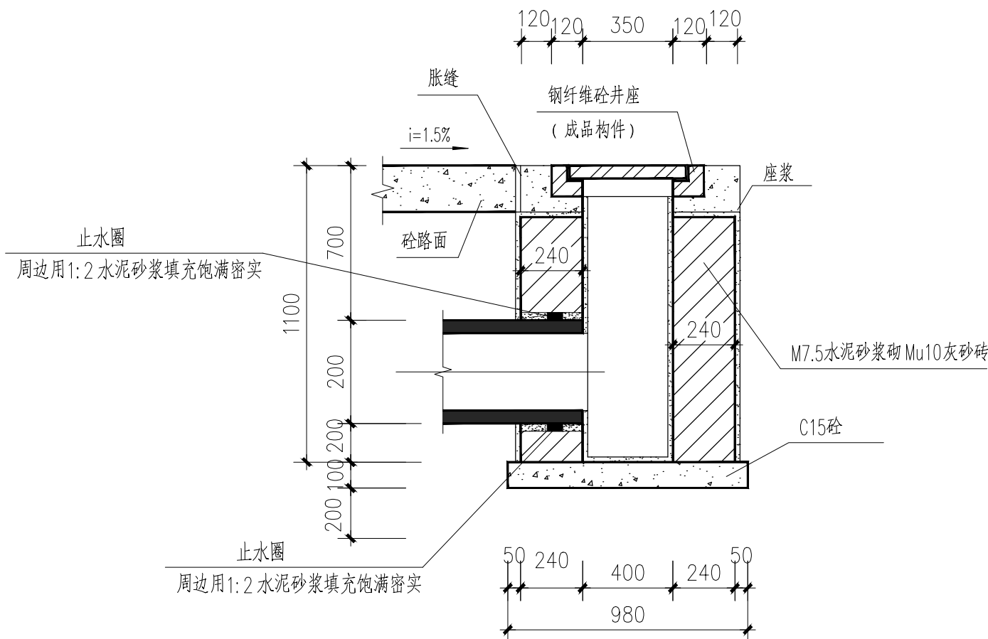
2-2剖面
