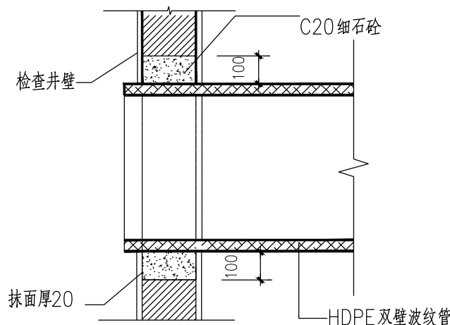
管道与检查井的连接大样
