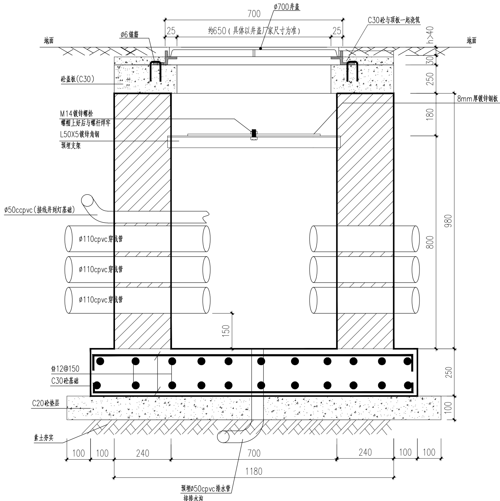
A-A剖面
