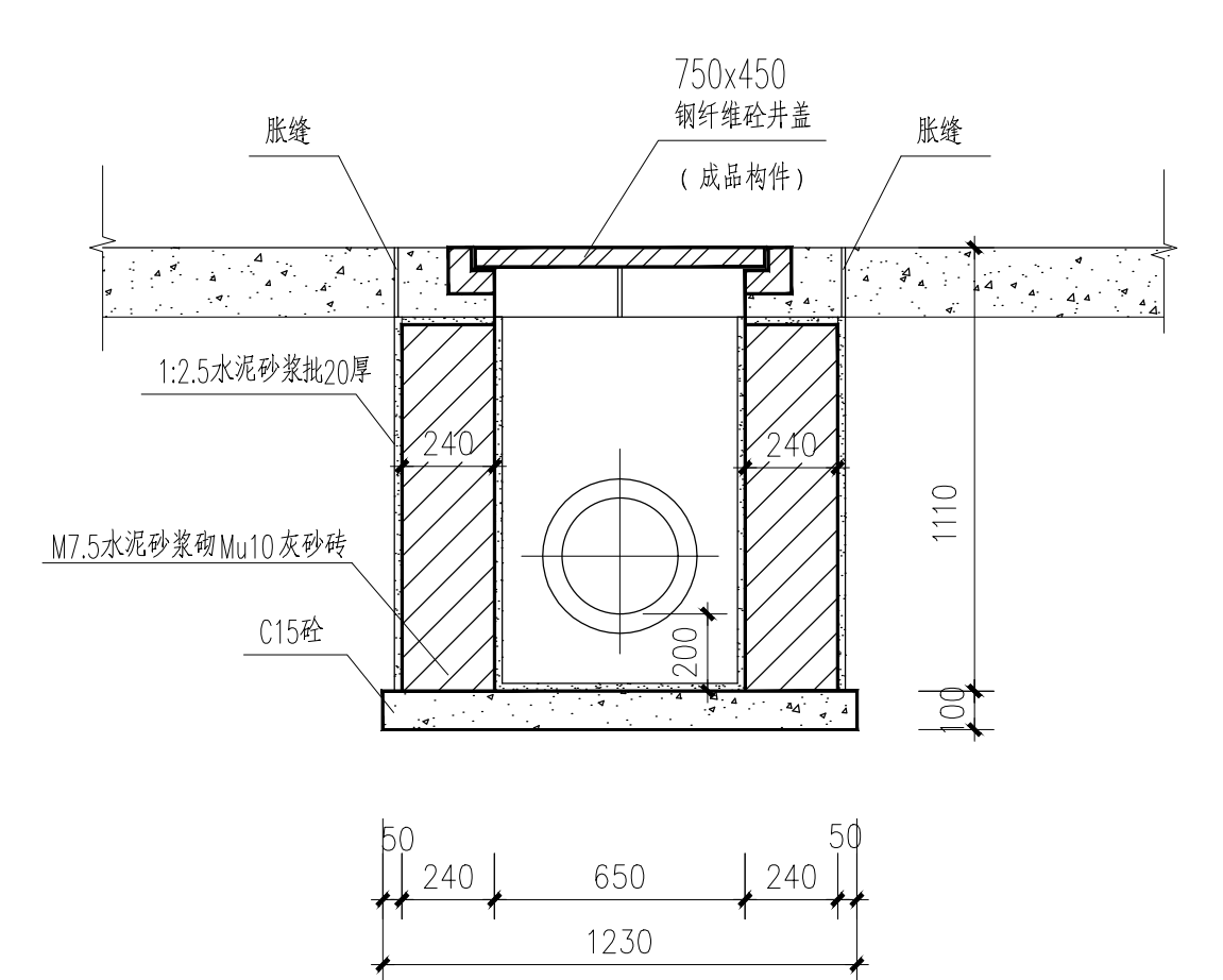
1-1剖面
