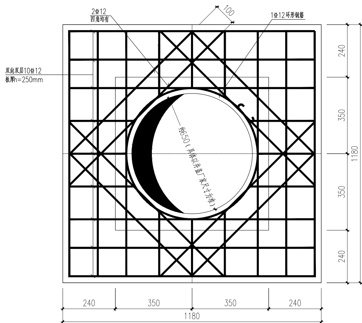
砼顶板配筋图
