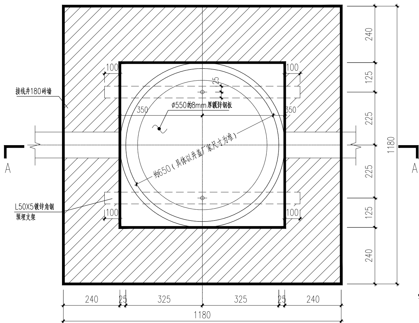
接线井平面图
