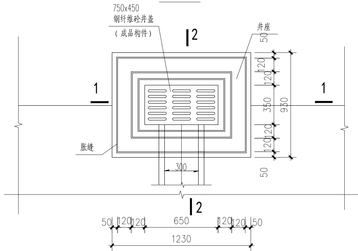
平面图
