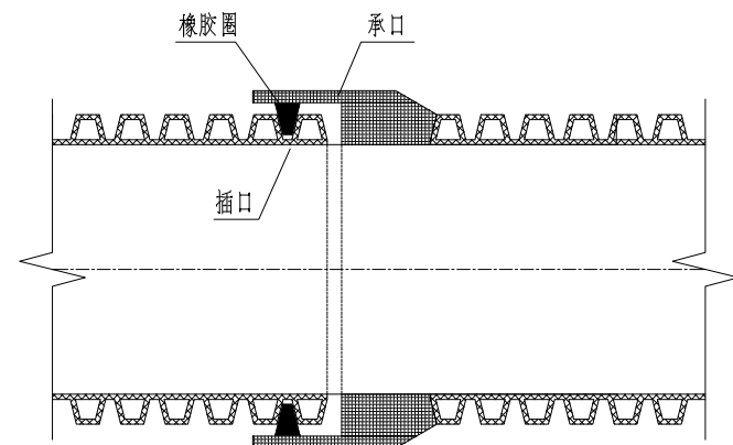
HDPE双壁波纹管连接示意图
