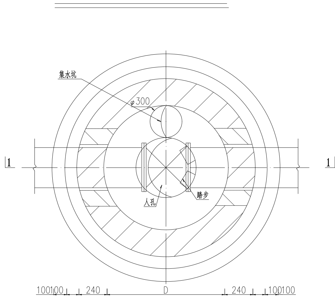
阀门井平面图
