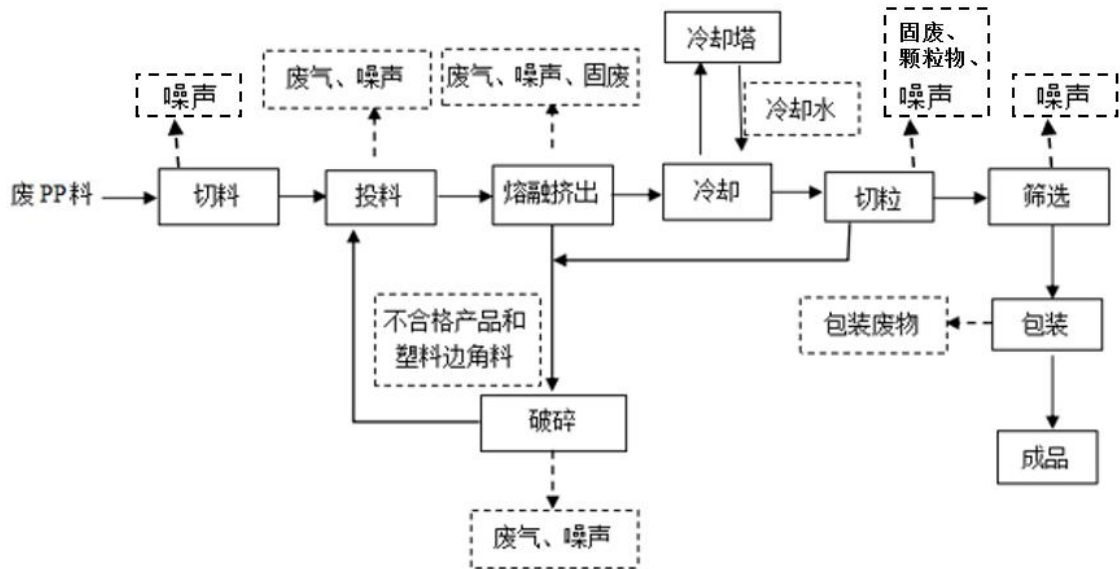
图 2-2 项目生产工艺流程及产排污环节图
