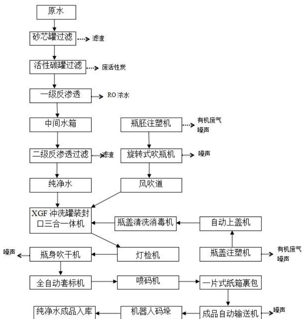
图2-8 瓶装饮用水生产工艺流程及产污环节图
