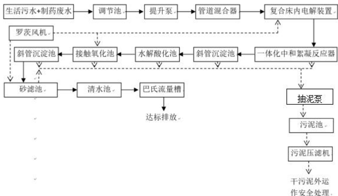
图 2-9 污水处理工艺流程图
