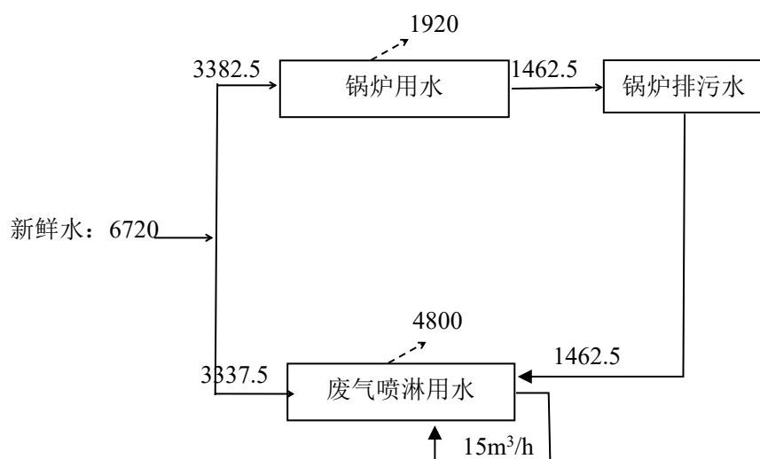
图 2-1 一期技改项目水平衡图 (单位: m³/a)
