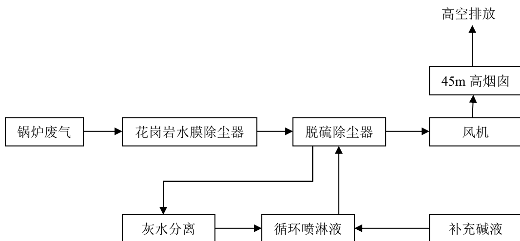
图 2-10 锅炉废气处理工艺流程图
