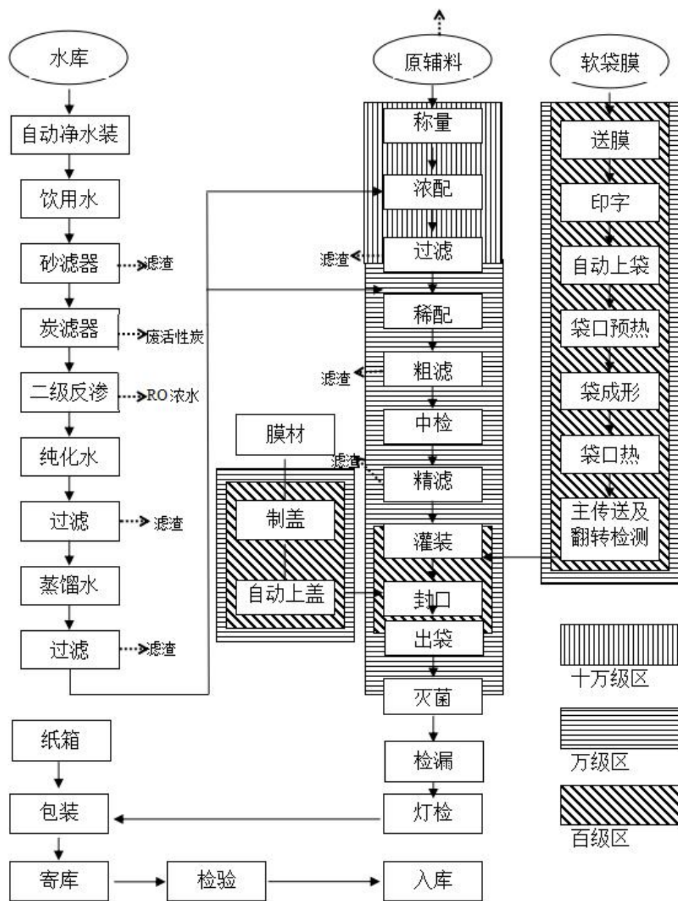
图2-7 非PVC软袋输液生产工艺流程及产污环节图
