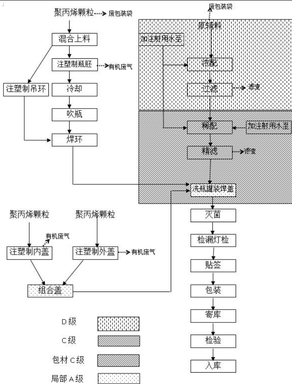
图 2-6 塑料瓶包装输液生产工艺流程及产污环节图
