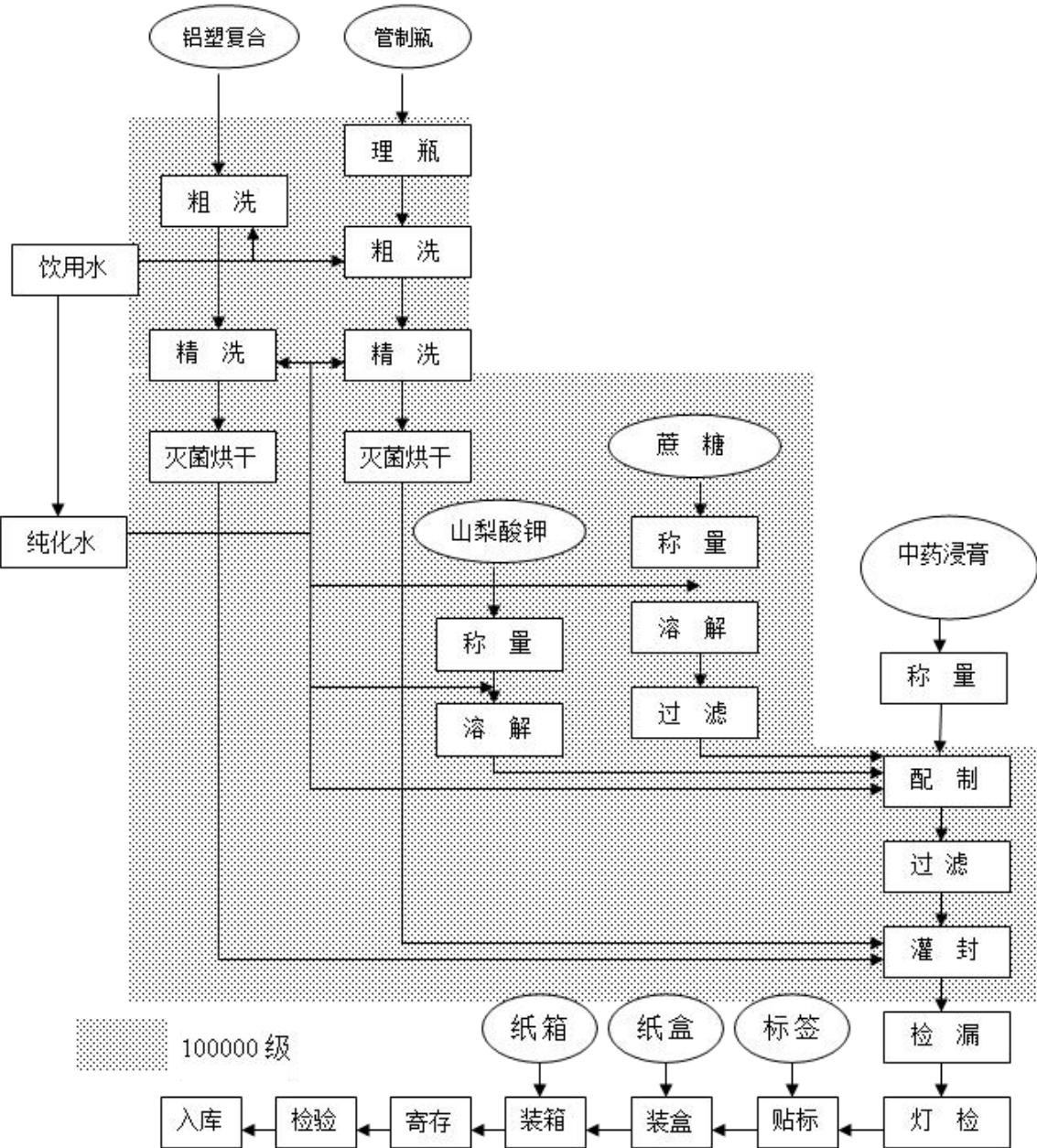
图 2-4 口服液生产工艺流程及产污环节图
