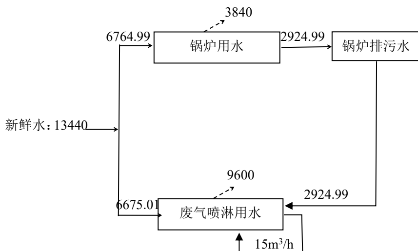
图 2-2 二期技改后项目水平衡图 (单位: m³/a)
