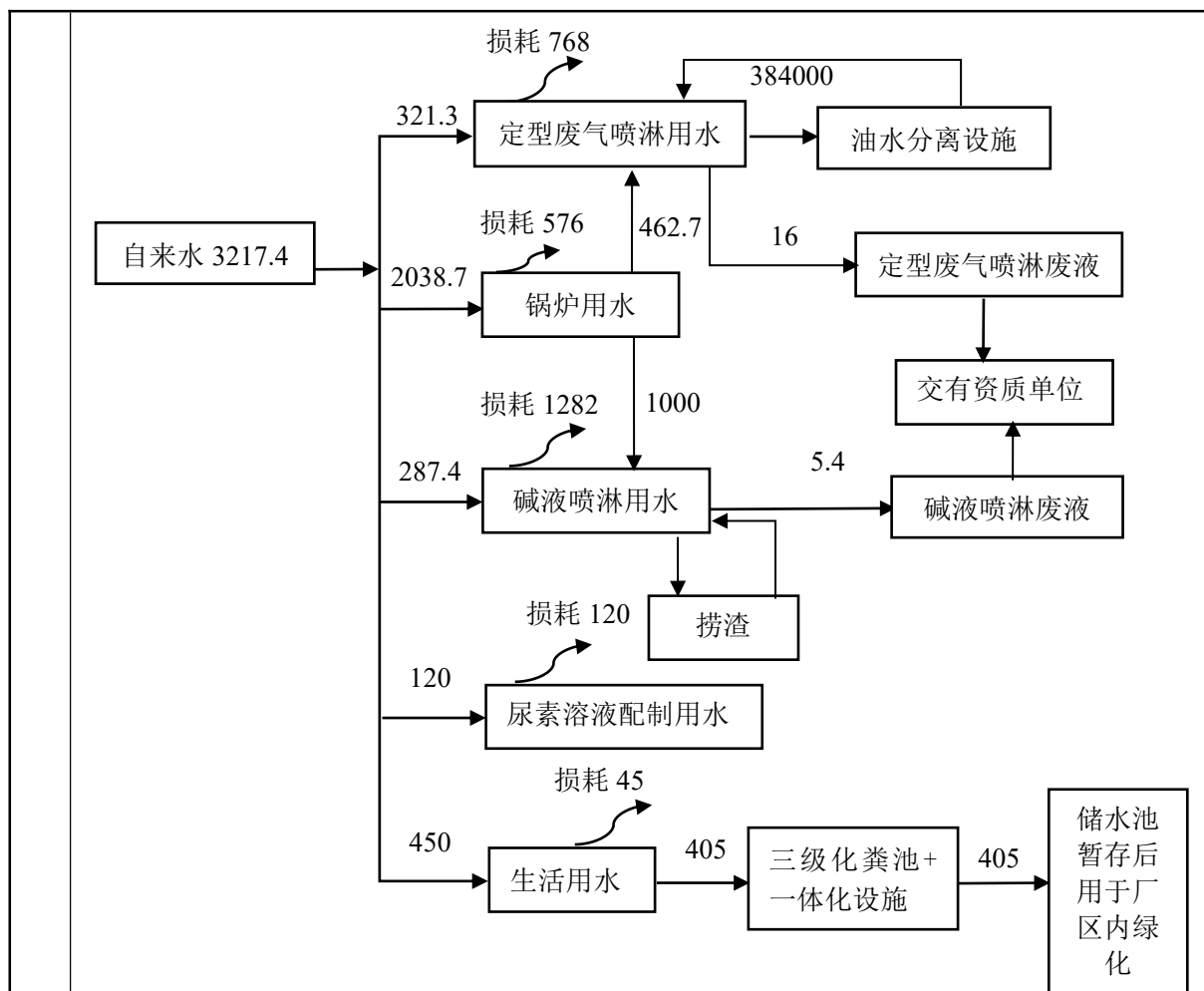
图 2-1 项目厂区水平衡图 (t/a)
