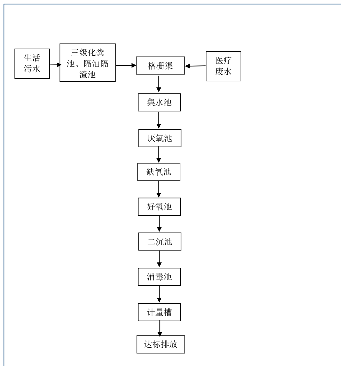
图 6.1-1 项目污水处理工艺流程图
