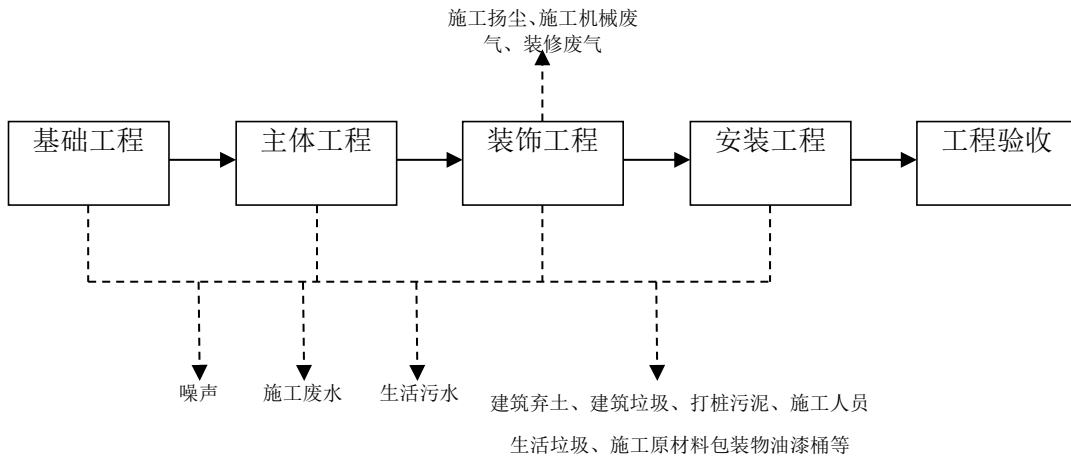
图 2-2 施工期作业流程图
