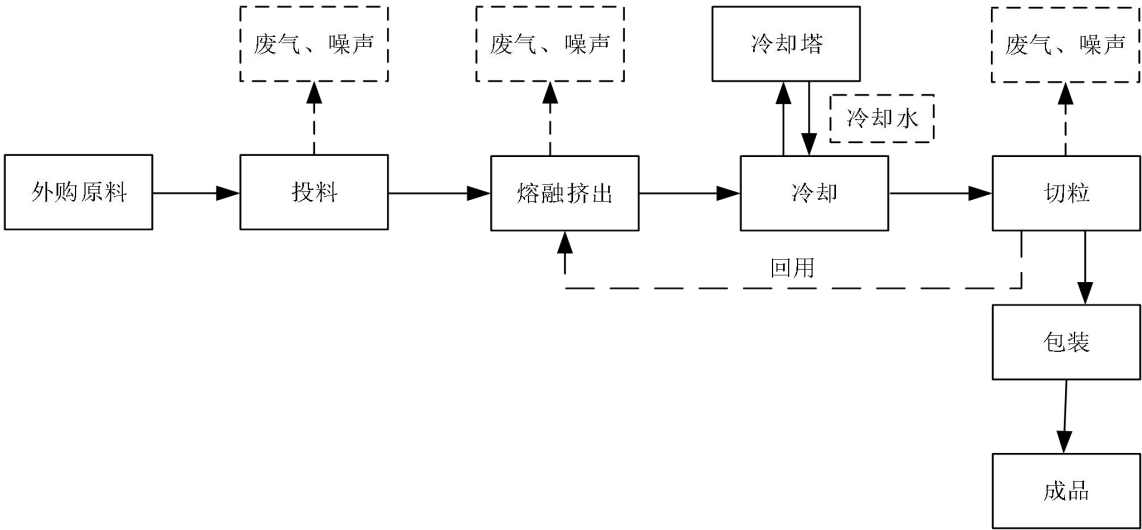
图 2-2 项目生产工艺流程图
