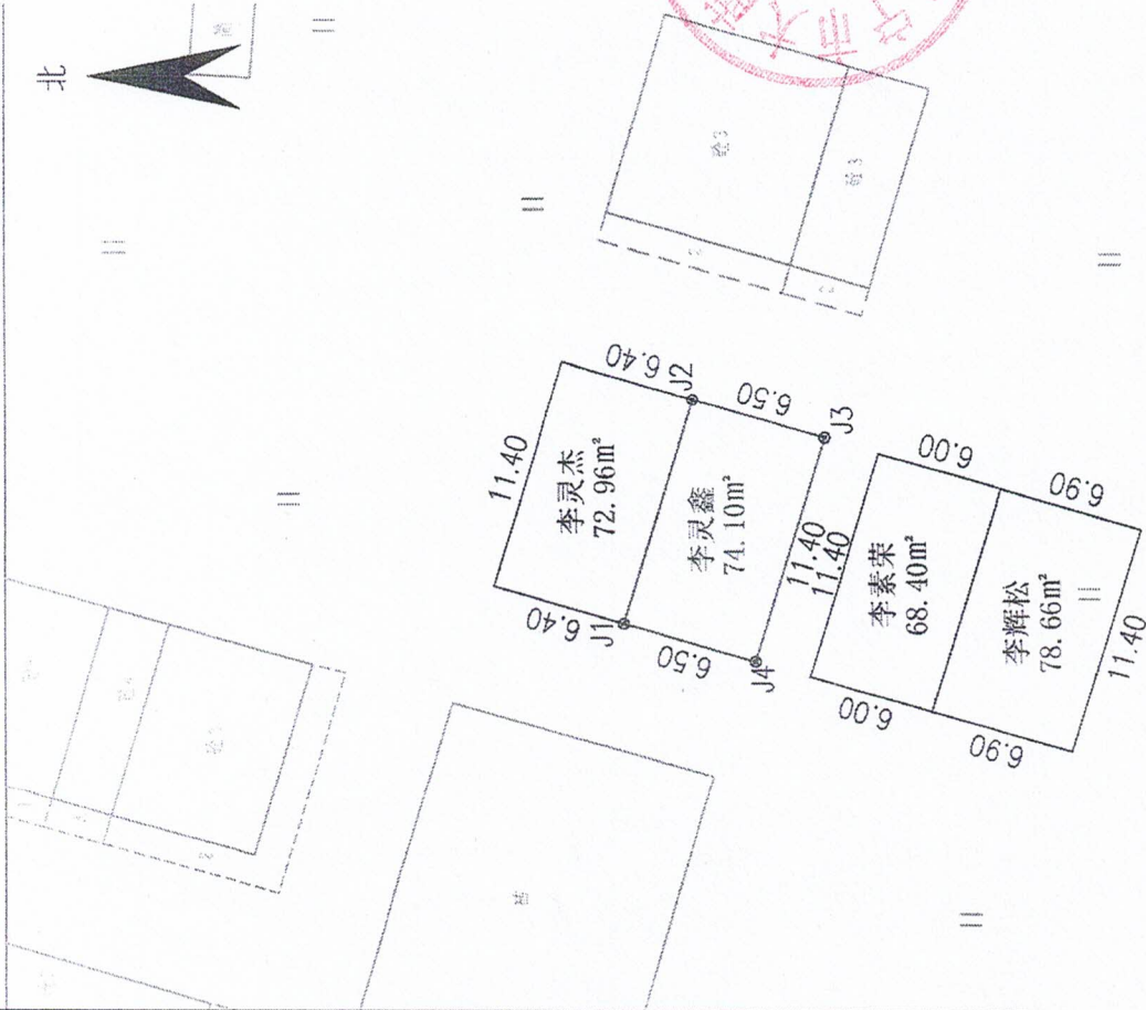
李灵鑫宅基地坐落平面位置图
