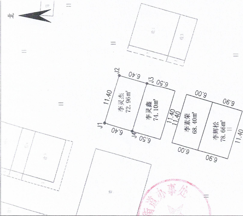
普宁市大南山街道和美村民宅基地平面图
