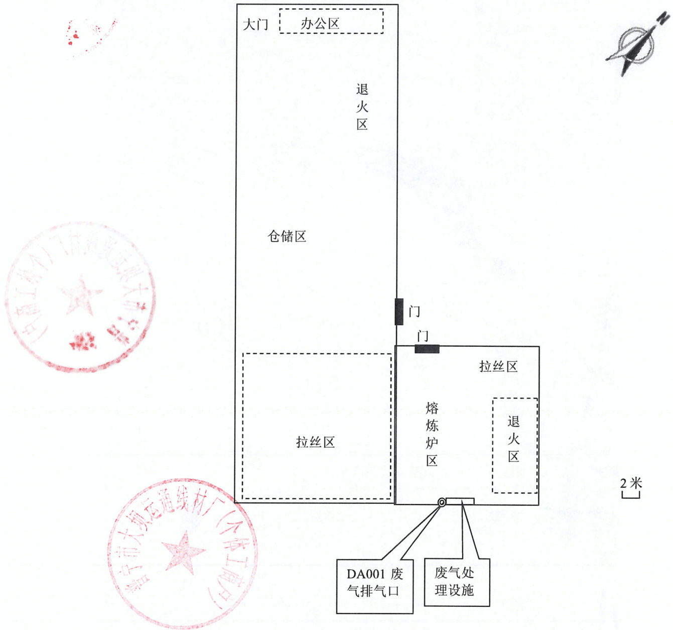
附图 2 项目平面布置图
