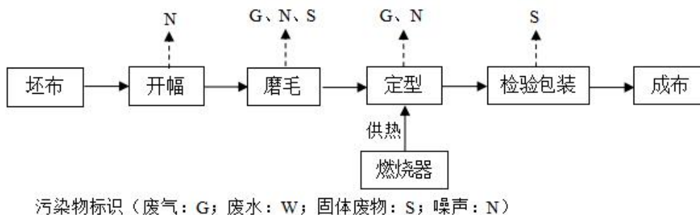
图 2-3 现有项目运行工艺流程及产污环节图
