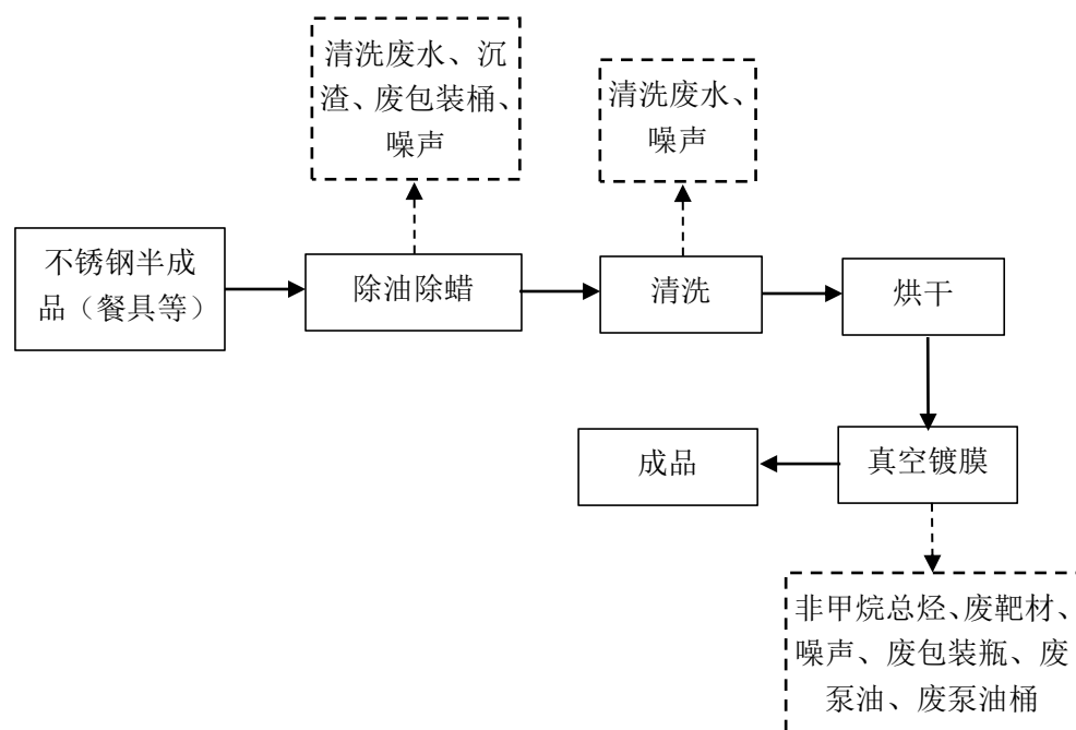
图 2-2 工艺流程图
