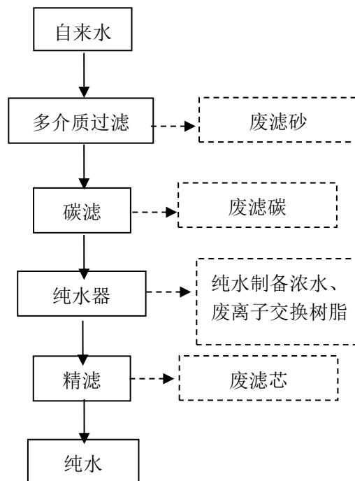
图 2-3 纯水制备工艺流程图
