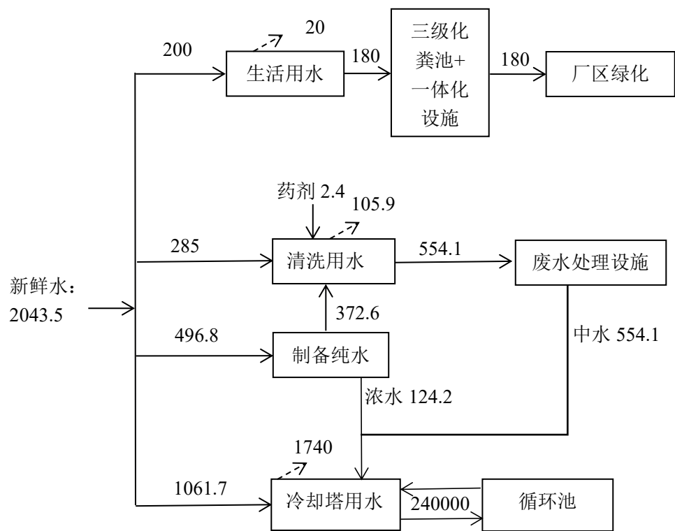
项目水平衡见图 2-1。
