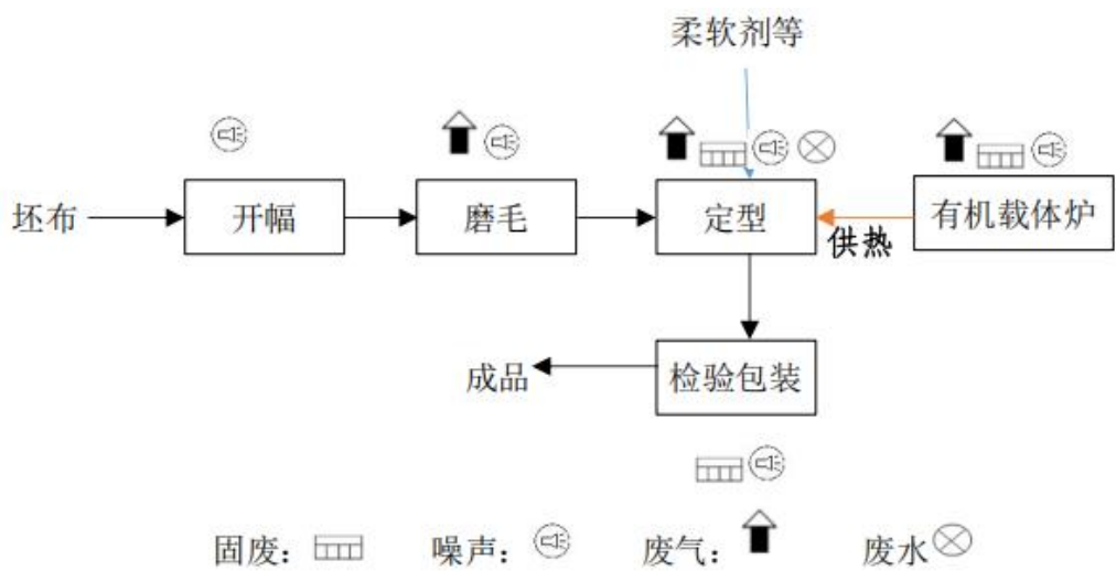
图 2-3 项目运行工艺流程及产污环节图
