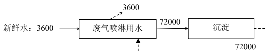
图 2-1 改建项目水平衡图（单位：m 3 /a）
