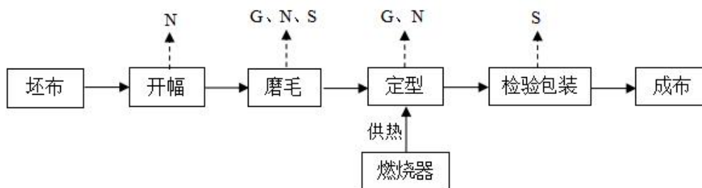
图 2-3 现有项目运行工艺流程及产污环节图
