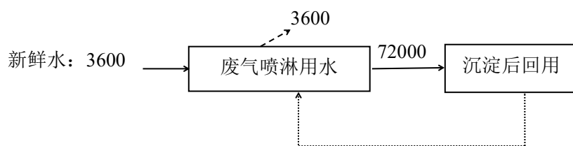
图 2-1 改建项目水平衡图（单位： \text{m}^3/\text{a} ）
