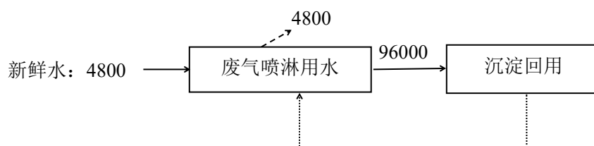
图 2-1 改建项目水平衡图（单位：m 3 /a）
