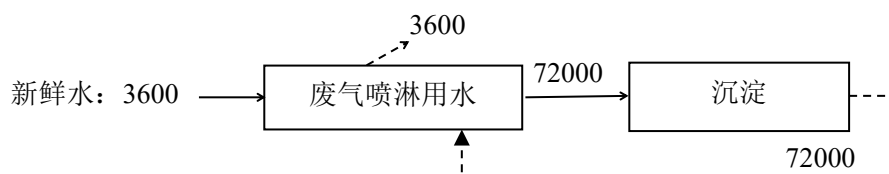
图 2-1 改建项目水平衡图（单位：m 3 /a）
