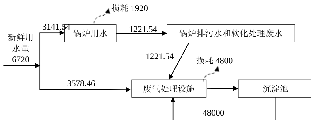
图 2-1 改建项目水平衡图 (单位: m³/a)
