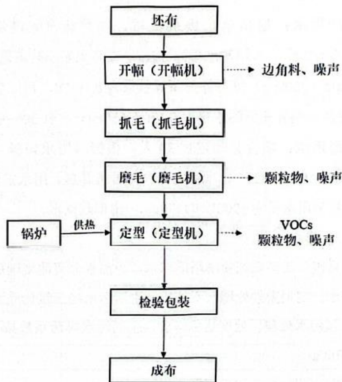
图 2-3 项目运行工艺流程及产污环节图
