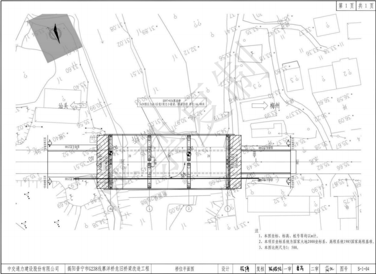
附图 11 项目平面、立面布置图
