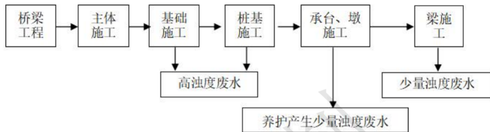
图 4-1 桥梁施工工艺及产物环节示意图
