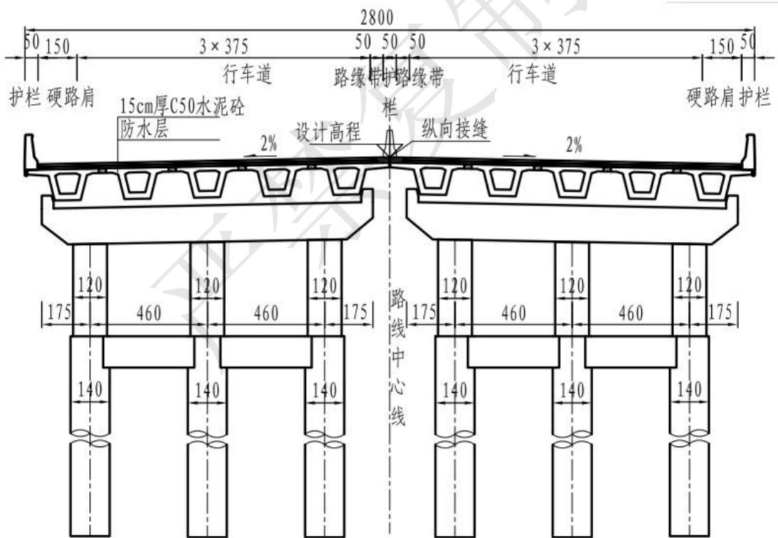
图 2-5 寨洋桥断面布置图
