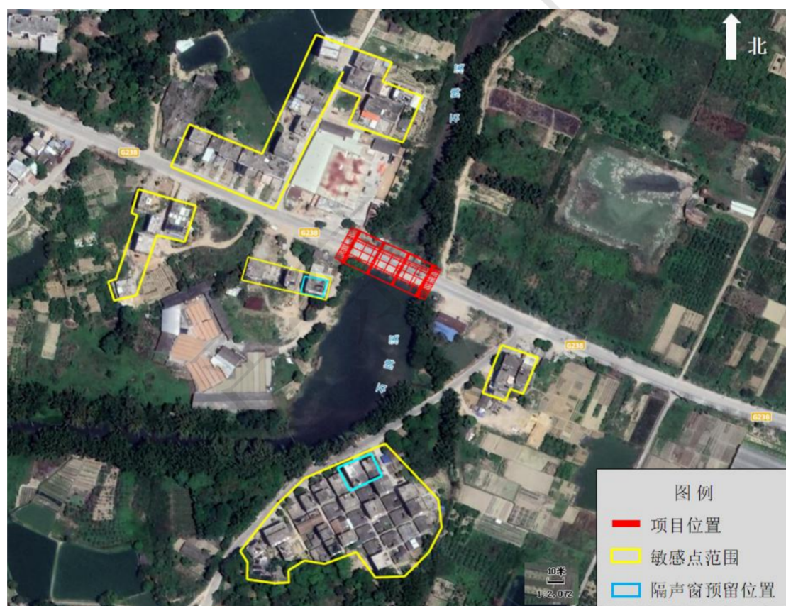
图 5.2-1 营运远期隔声窗预留位置
