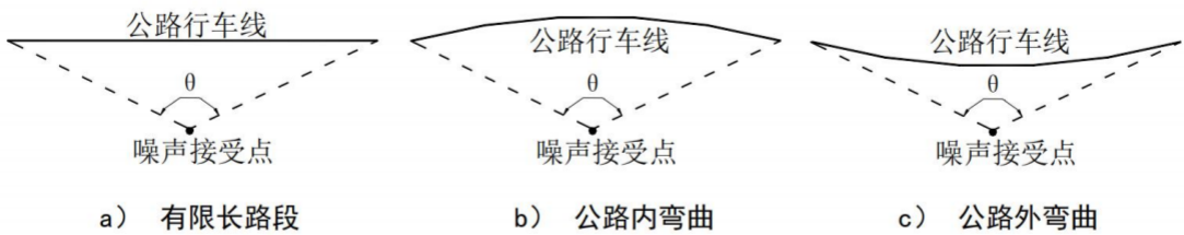
图 4.2-5 预测点到有限长路段两端的张角
