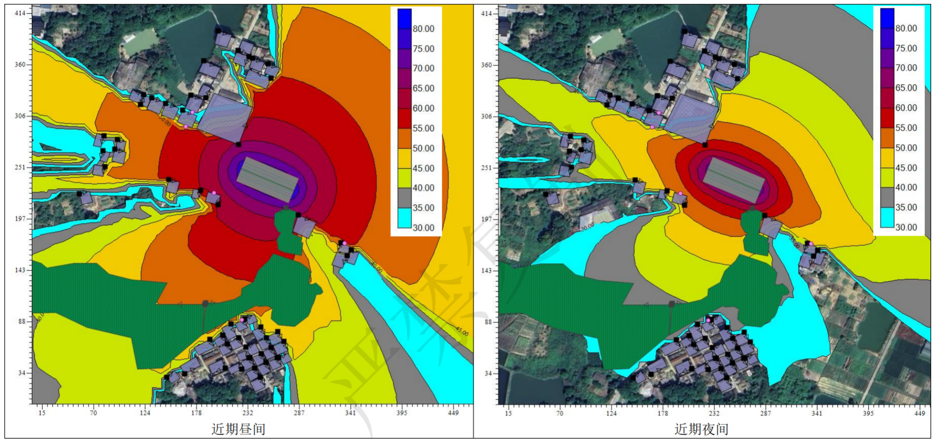
图 4.2-6 营运近期等声级线图
