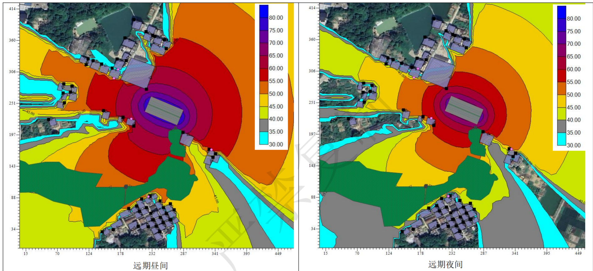
图 4.2-8 营运远期等声级线图
