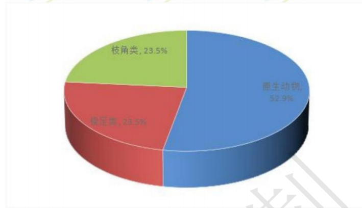
图 6.2-1 W1 寨洋桥浮游动物种类组成图
