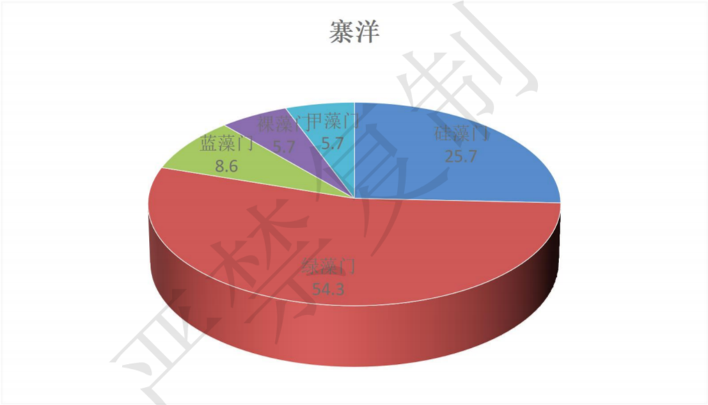
图 3-1 寨洋浮游植物种类组成图
