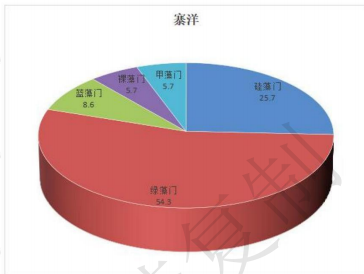
图 6.1-1 寨洋浮游植物种类组成图
