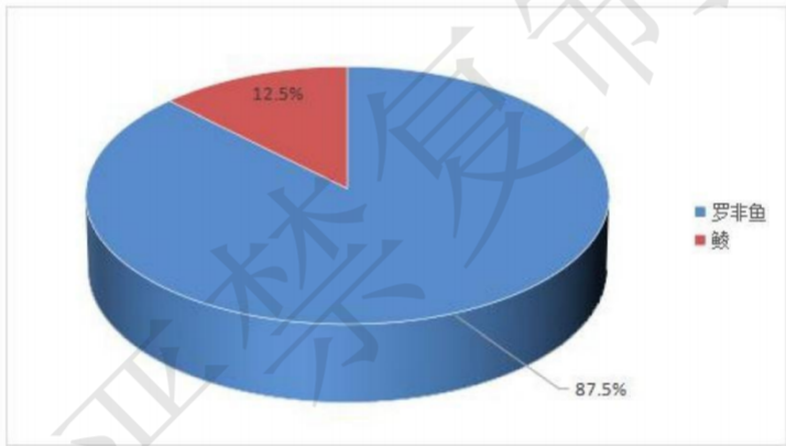
图 6.4-1 W1 寨洋桥调查断面鱼类种类组成图
