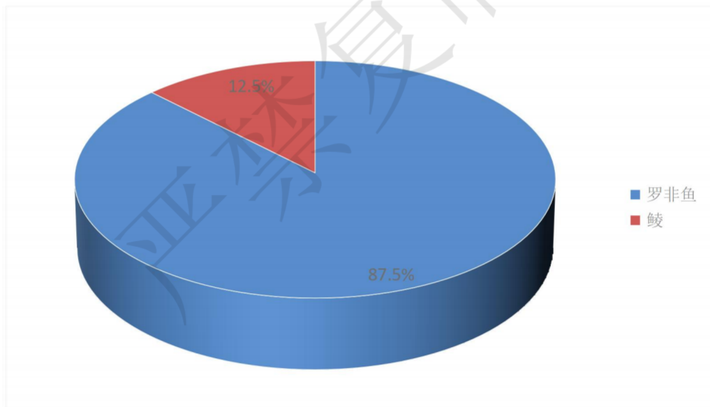
图 3-7 W1 寨洋调查断面鱼类种类组成图
