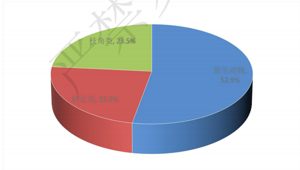
图 3-3 W1 寨洋浮游动物种类组成图
