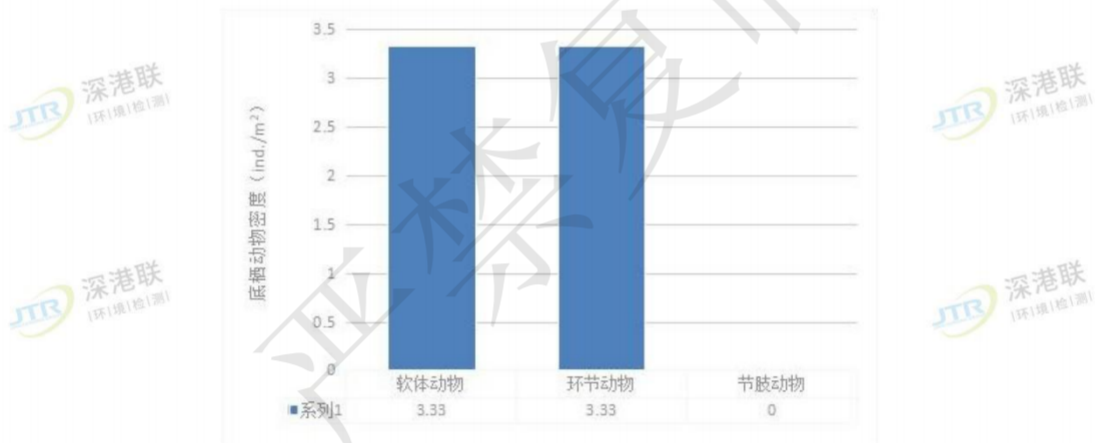
图 6.3-2 底栖动物栖息密度分布图（单位： \text{ind./m}^2 ）
