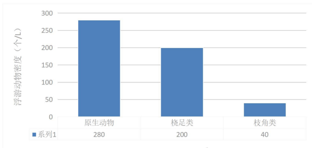
图 3-4 W1 寨洋浮游动物各门类密度的分布图（单位：个/L）
