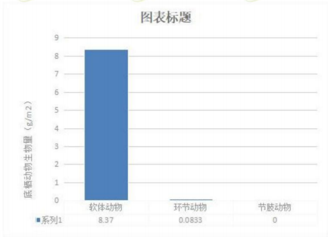
图 6.3-3 底栖动物生物量分布图 (单位: g/m 2 )
