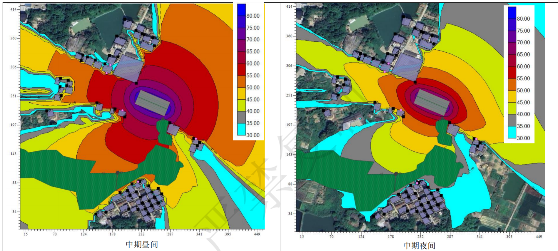
图 4.2-7 营运中期等声级线图
