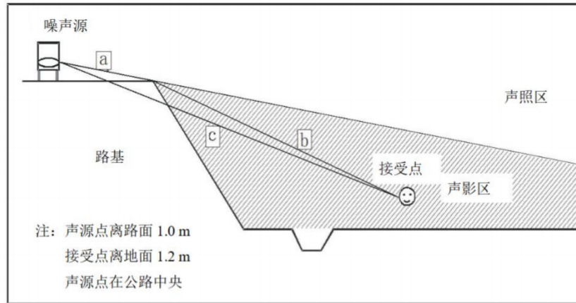
图 4.2-1 声程差 \delta 计算示意图
