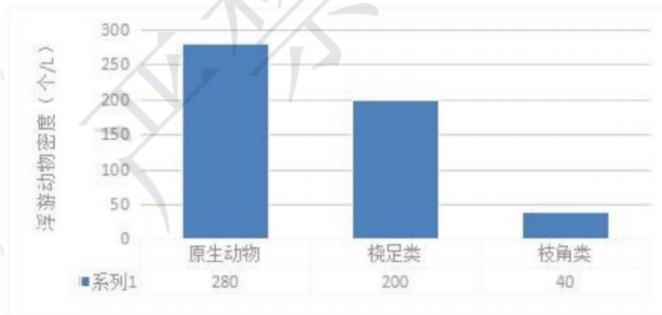
图 6.2-2 W1 寨洋桥浮游动物各门类密度的分布图 (单位: 个/L)
