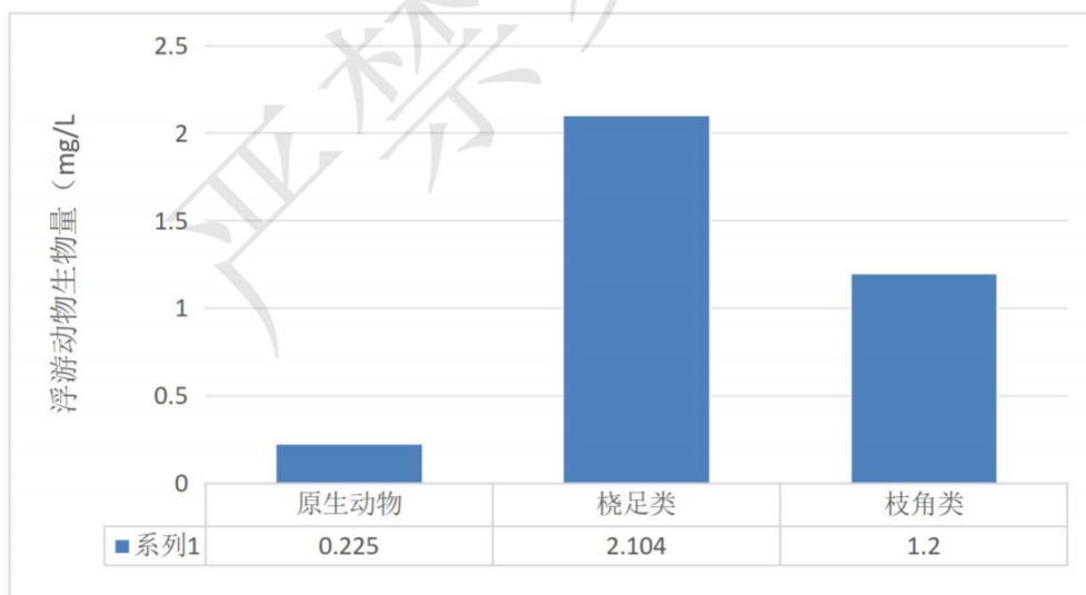
图 3-5 W1 寨洋断面浮游动物生物量分布图（单位：mg/L）
