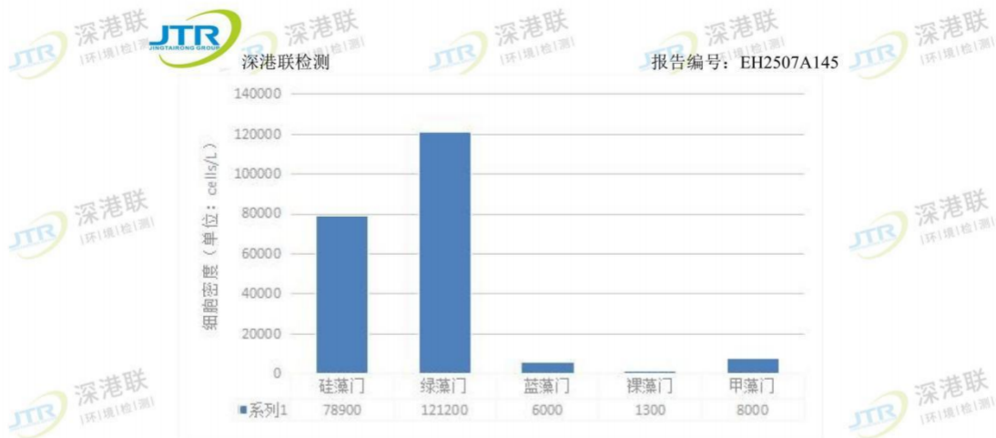
图 6.1-2 W1 寨洋桥断面浮游植物细胞各门细胞密度分布图 (单位: cells/L)
