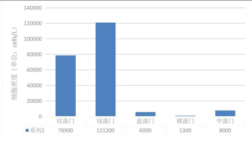
图 3-2 W1 寨洋断面浮游植物细胞各门细胞密度分布图 (单位: cells/L)
