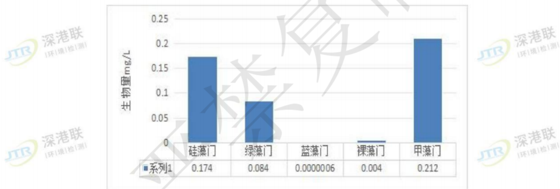
图 6.1-3 W1 断面浮游植物生物量分布图 (单位: mg/L)
