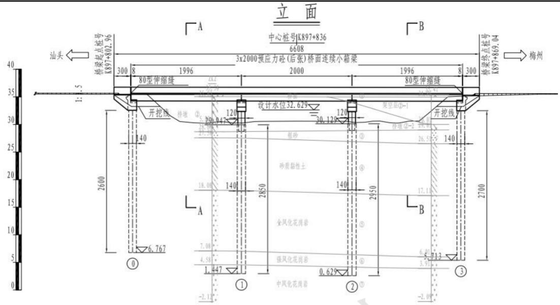
图 2-4 寨洋桥立面设计图
