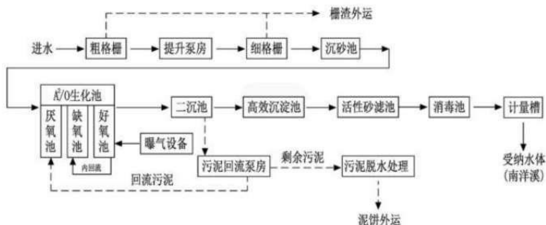
图 4-2 普宁市南径镇污水处理厂污水处理工艺
