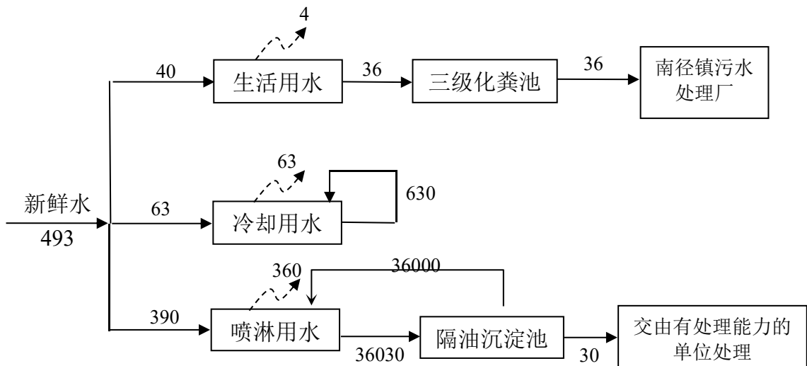
图 2-1 项目水平衡图（单位：m³/a）
