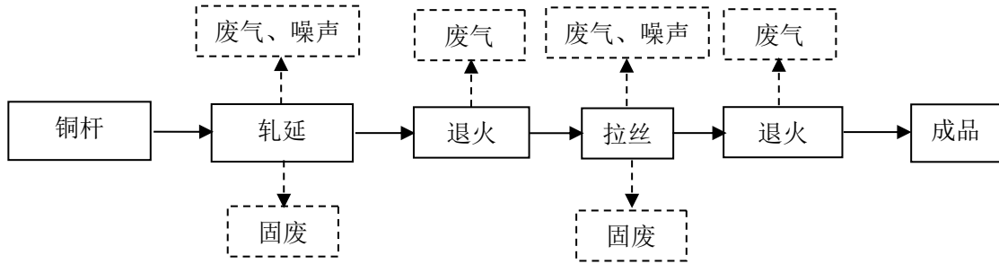
图 2-2 项目生产工艺流程及产排污环节图
