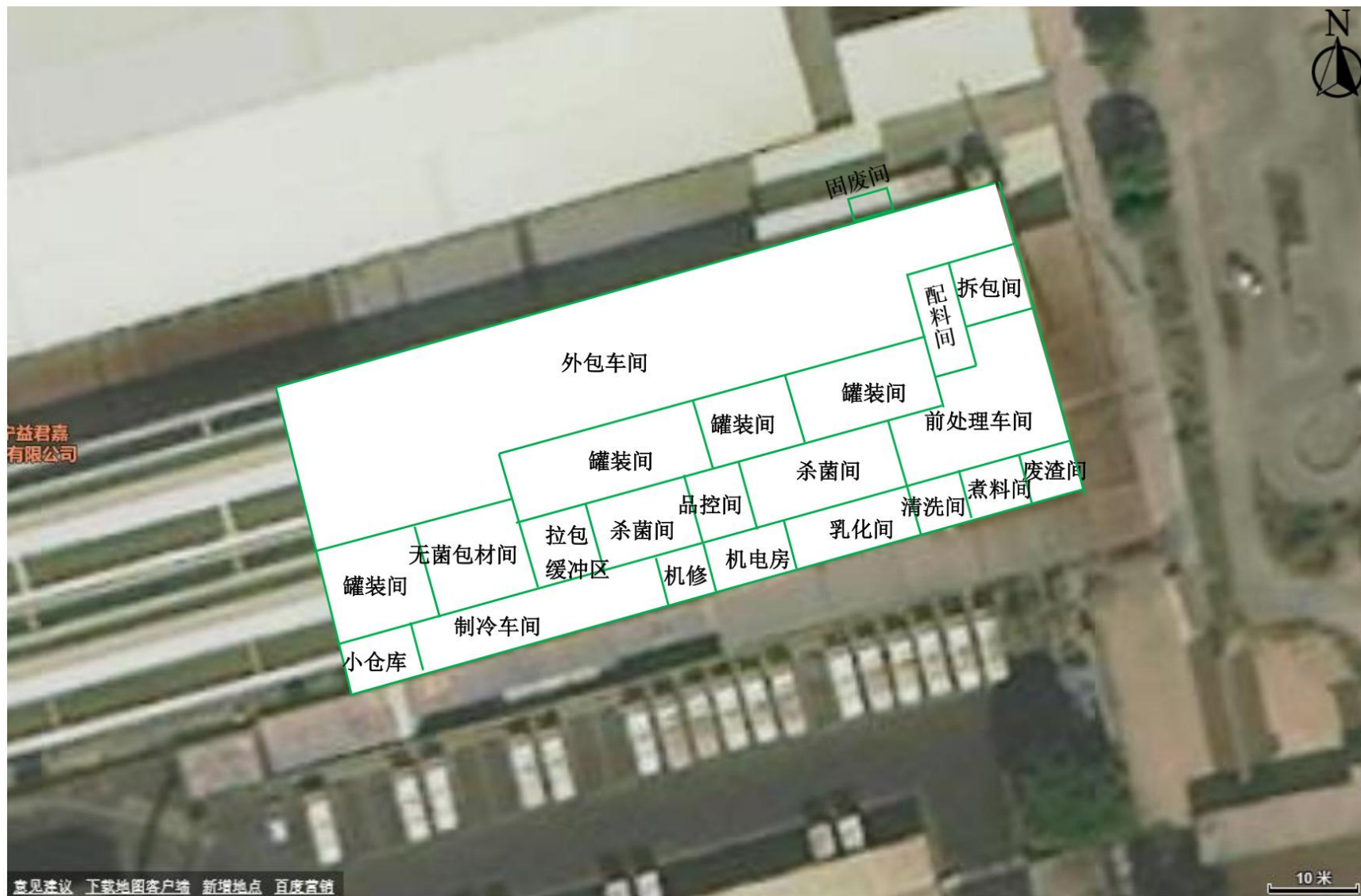
附图 4-2 项目平面布置图
