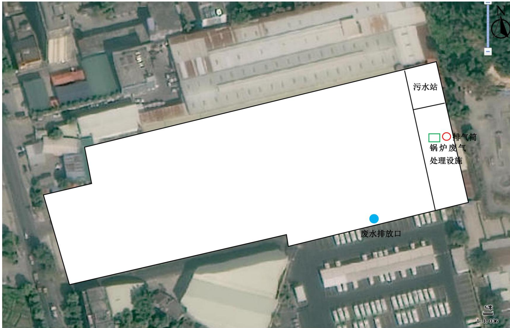
附图 4-4 项目平面布置图（排气筒、排水口、处理设施等位置）
