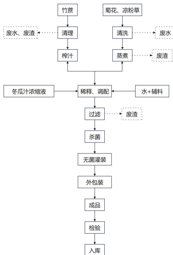
图 2-2 菊花茶等各类饮料工艺流程图
