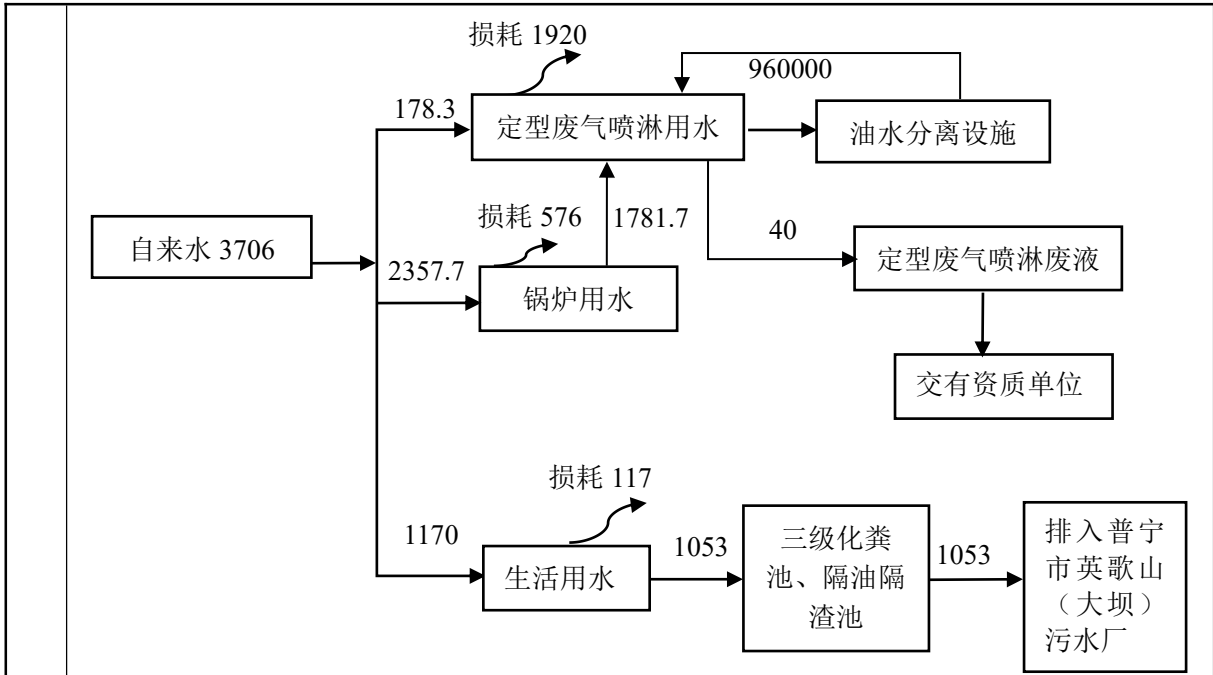
图 2-1 项目厂区水平衡图 (t/a)
