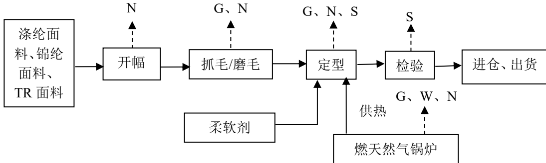
图 2-2 项目运营期流程
