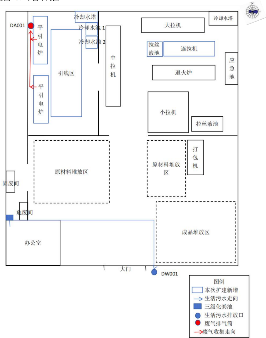
附图 10：平面布局图
