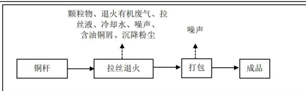
图 2-3 现有项目生产工艺流程图
