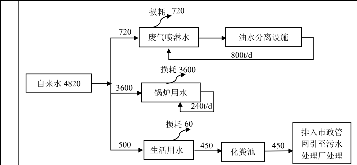
图 2-1 项目厂区水平衡图 (t/a)
