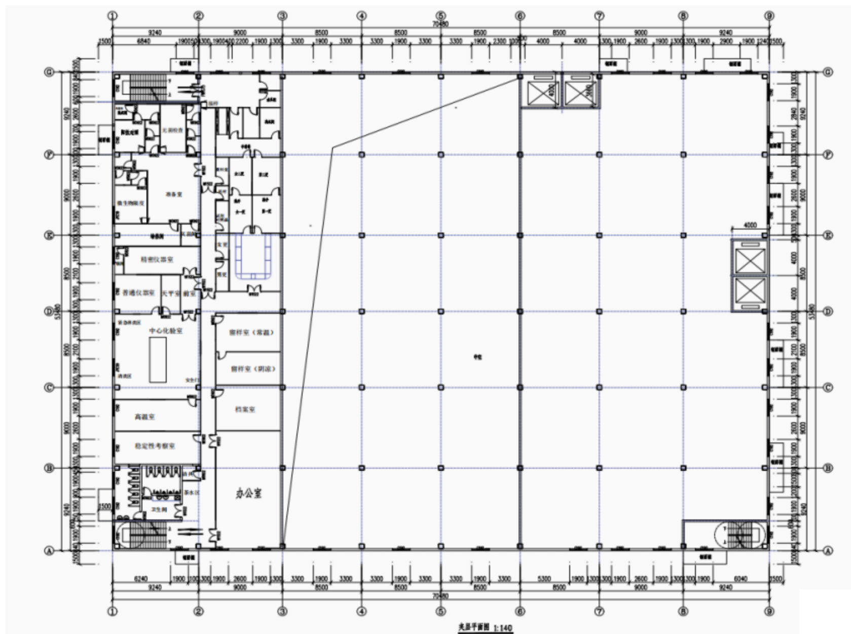
附图7 厂区平面布置图 (夹层)
